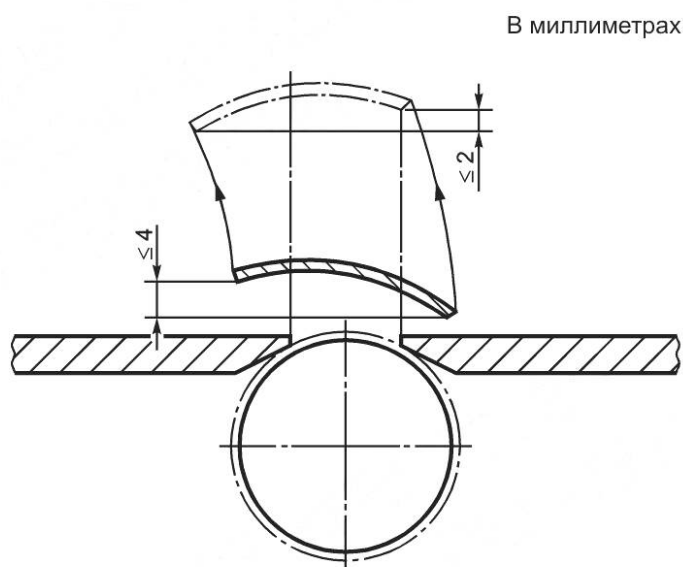
Рисунок 8 — Пример защитного ограждения мостового типа
