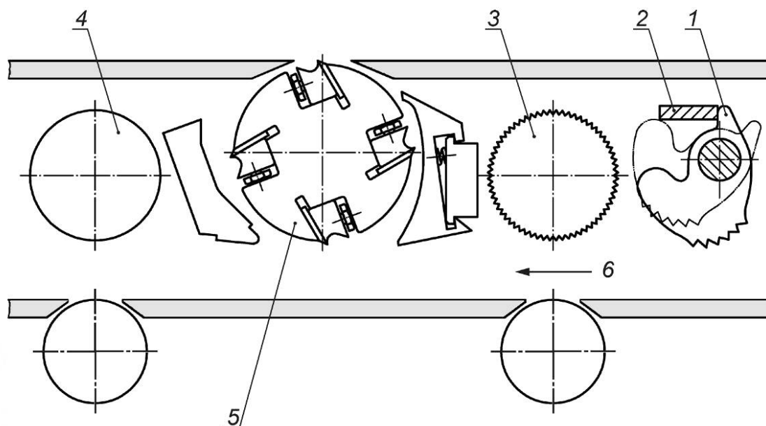
1 — устройство, предотвращающее обратный удар; 2 — стопор от вращения устройства от обратного удара; 3 — подающий валец на входе; 4 — приемный валец на выходе; 5 — ножевой вал; 6 — направление подачи
