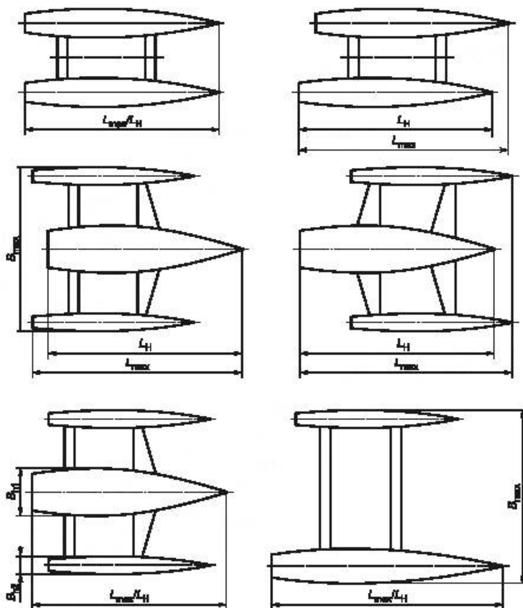
Рисунок 2 — Определение L_{\text{max}} , L_H , B_{\text{max}} и B_H для многокорпусных судов
