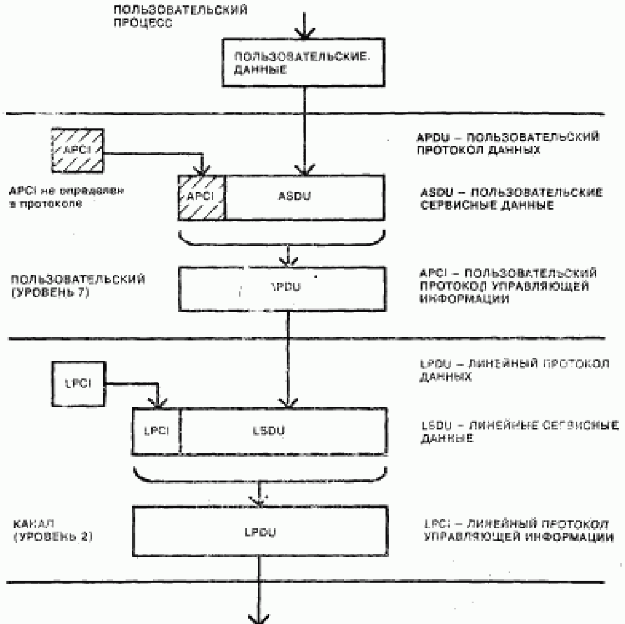
Рисунок 4 — Связи между блоками данных
