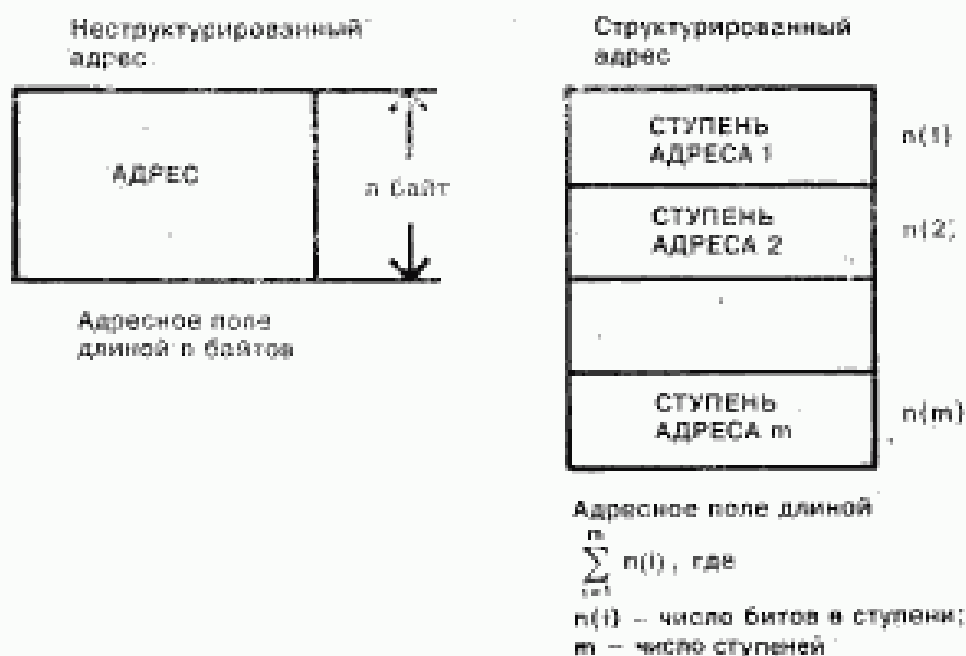
Рисунок 10 — Два типа адресов ОБЪЕКТОВ ИНФОРМАЦИИ
