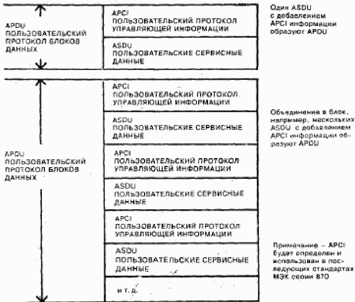
Рисунок 5 — Общая структура ПОЛЬЗОВАТЕЛЬСКОГО ПРОТОКОЛА БЛОКОВ ДАННЫХ
