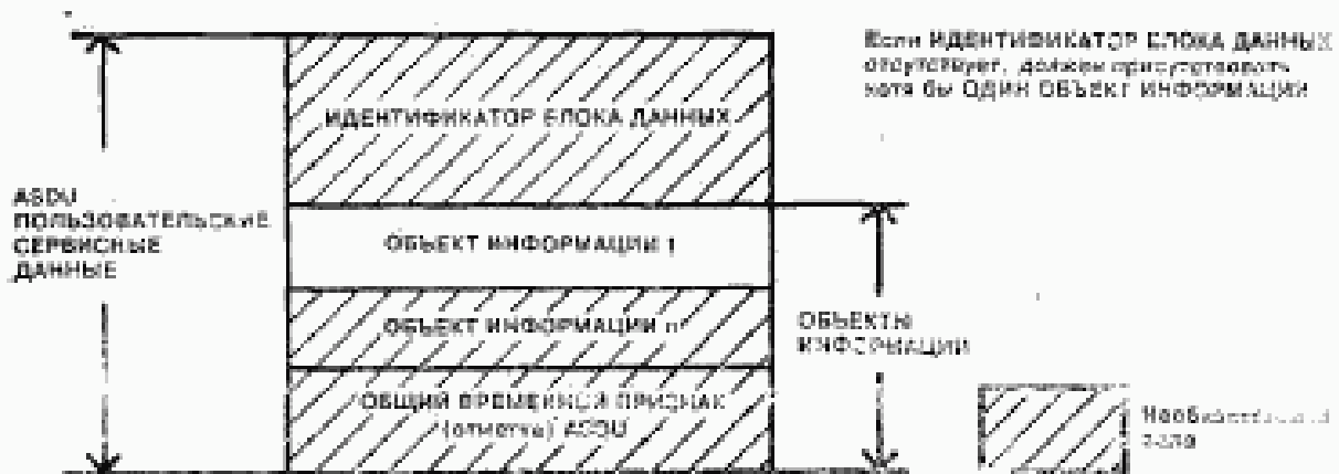
Рисунок 6 — Основная структура БЛОКА ПОЛЬЗОВАТЕЛЬСКИХ СЕРВИСНЫХ ДАННЫХ
