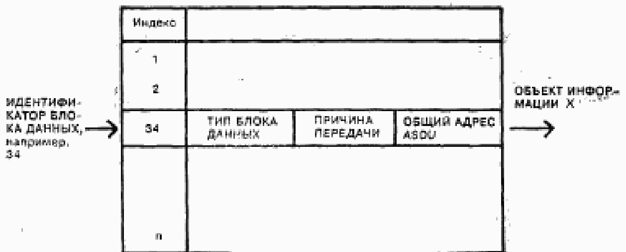
Рисунок 9 — Пример компактной идентификации ОБЪЕКТОВ ИНФОРМАЦИИ
