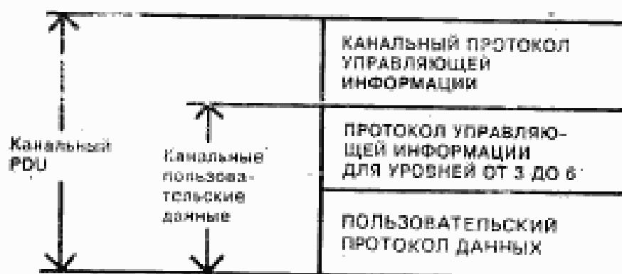
Рисунок 2 — Структура кадра для модели 1
