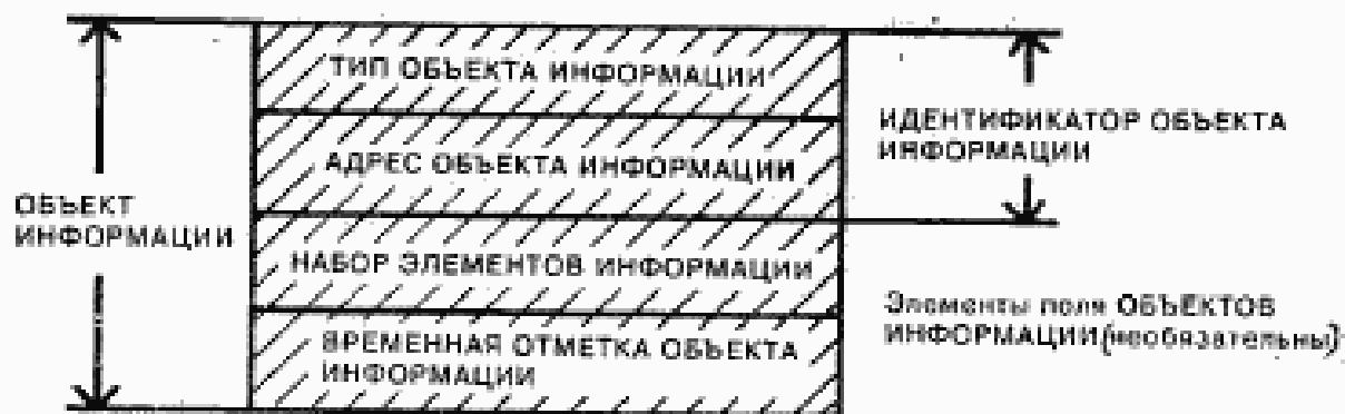
Рисунок 8 — Общая структура ОБЪЕКТА ИНФОРМАЦИИ
