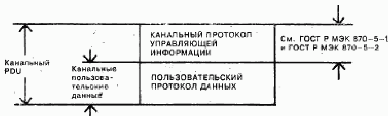
Рисунок 3 — Структура кадра для модели 2
