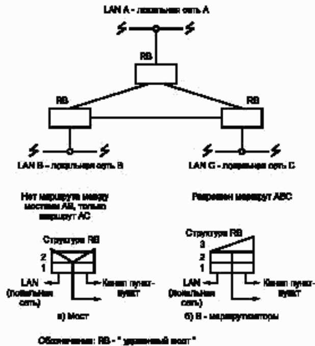
Рисунок 10 — Базовая структура с «удаленными мостами»
