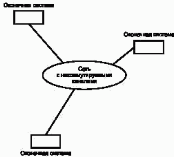
Рисунок 9 — Базовая структура, основанная на «некоммутируемых каналах»
