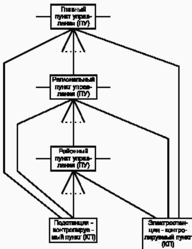
Рисунок 1 — Основная структура системы управления
