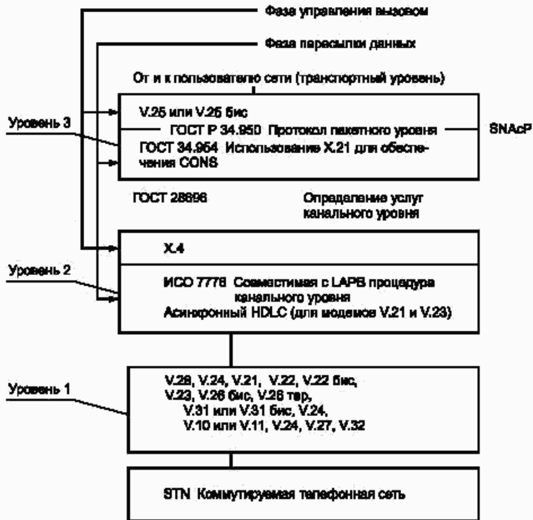
Рисунок 6 — Описание модели коммутируемой телефонной сети
