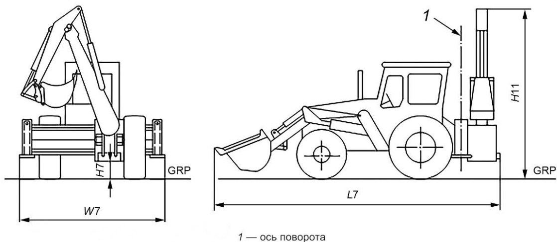
Рисунок 7 с) — Обратная лопата с боковым перемещением стрелы
