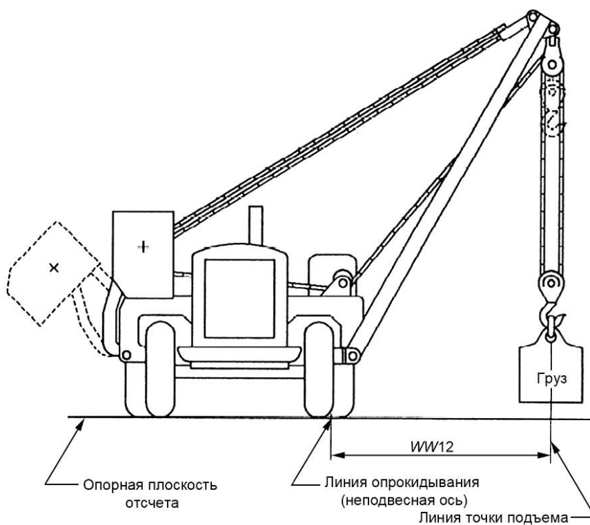
Рисунок 2 — Колесная машина с колесами в прямолинейном положении
