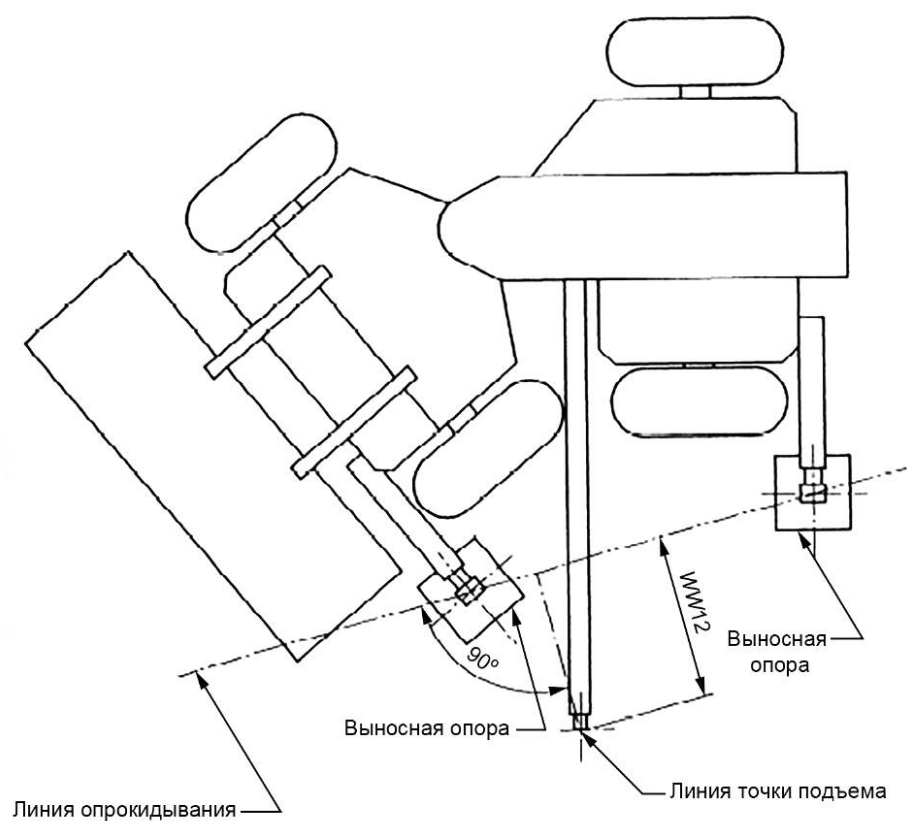
Рисунок 7 — Машина с шарнирно-сочлененной рамой в крайнем левом положении и с использованием выносных опор
