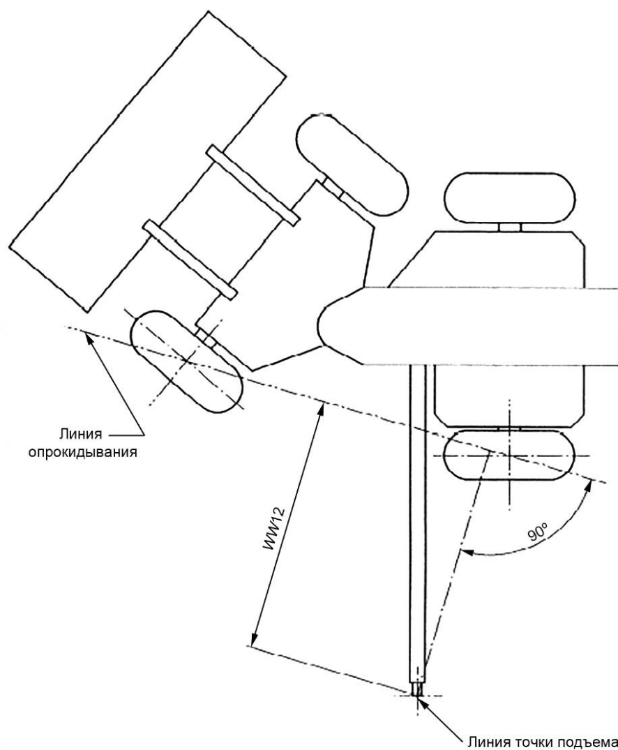
Рисунок 5 — Колесный трактор с шарнирно-сочлененной рамой в крайнем правом положении; с подвесной осью
