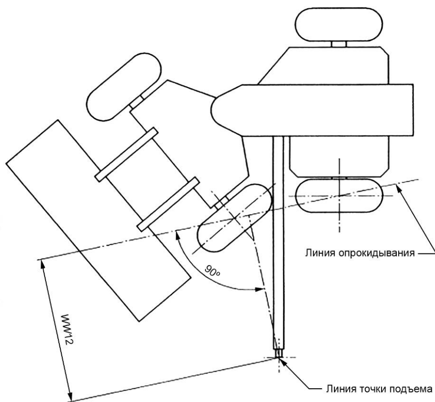
Рисунок 3 — Колесный трактор с шарнирно-сочлененной рамой в крайнем левом положении; с неподвесной осью
