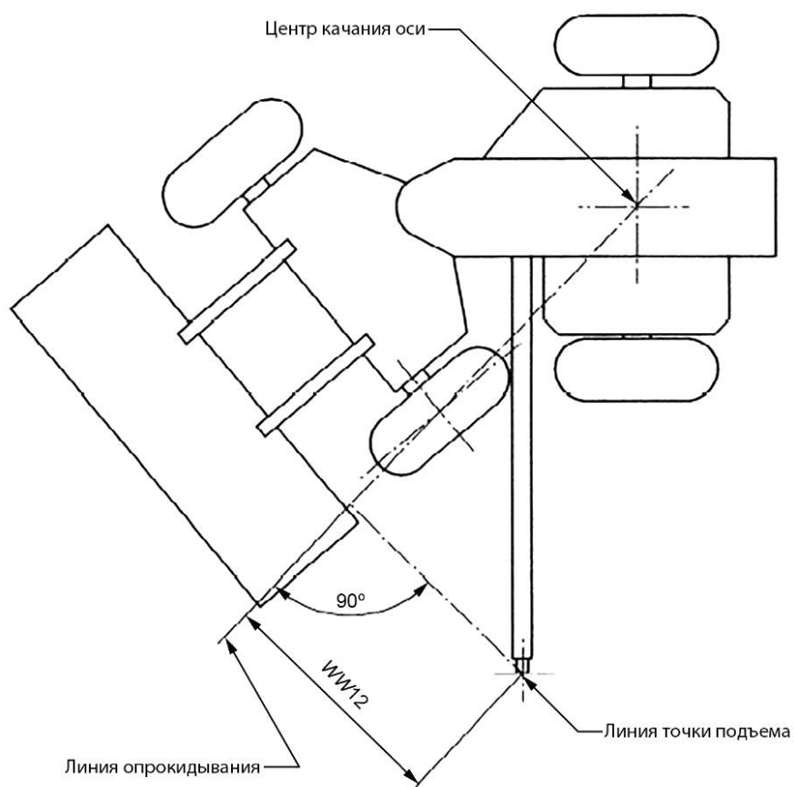
Рисунок 4 — Колесный трактор с шарнирно-сочлененной рамой в крайнем левом положении; с подвесной осью
