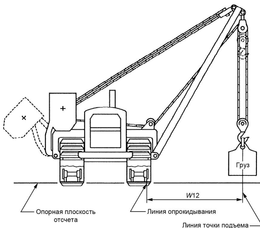
Рисунок 1 — Трубоукладчик
