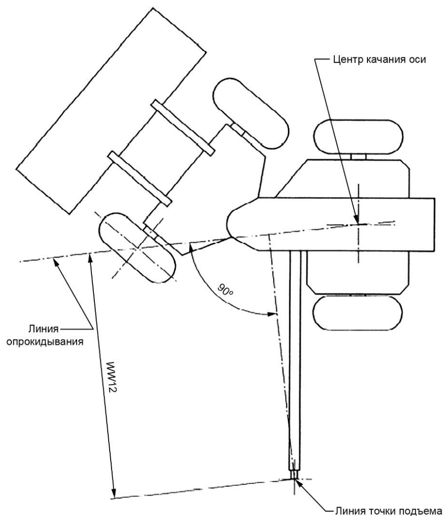
Рисунок 6 — Колесный трактор с шарнирно-сочлененной рамой в крайнем правом положении; с подвесной осью
