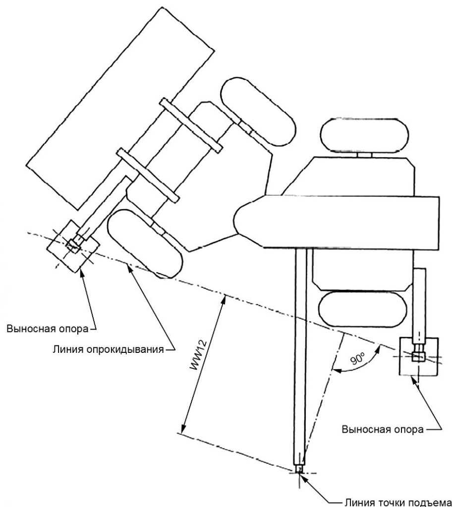
Рисунок 8 — Машина с шарнирно-сочлененной рамой в крайнем правом положении и с использованием выносных опор
