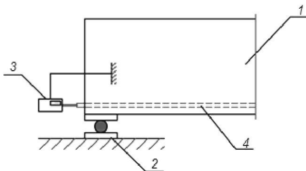
1 — изделие; 2 — шарнирно-подвижная опора; 3 — индикатор перемещений; 4 — арматурный стержень
