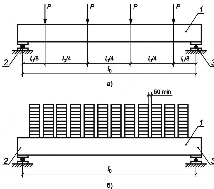
а) Сосредоточенными силами, эквивалентными равномерной нагрузке; б) Равномерно-распределенной нагрузкой штучными грузами; 1 — испытываемая конструкция; 2 — шарнирно-подвижная опора; 3 — шарнирно-неподвижная опора
