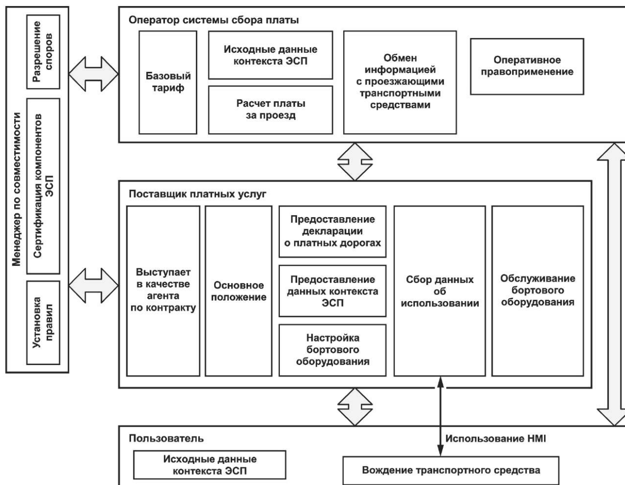
Рисунок 3 — Роли ЭСП, их обязанности и их взаимодействие
