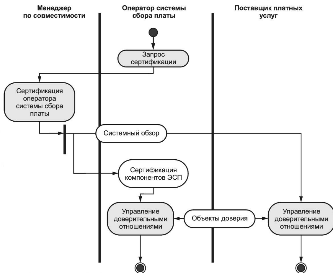
Рисунок 6 — Добавление/удаление нового оператора системы сбора платы в/из зоны совместимости
