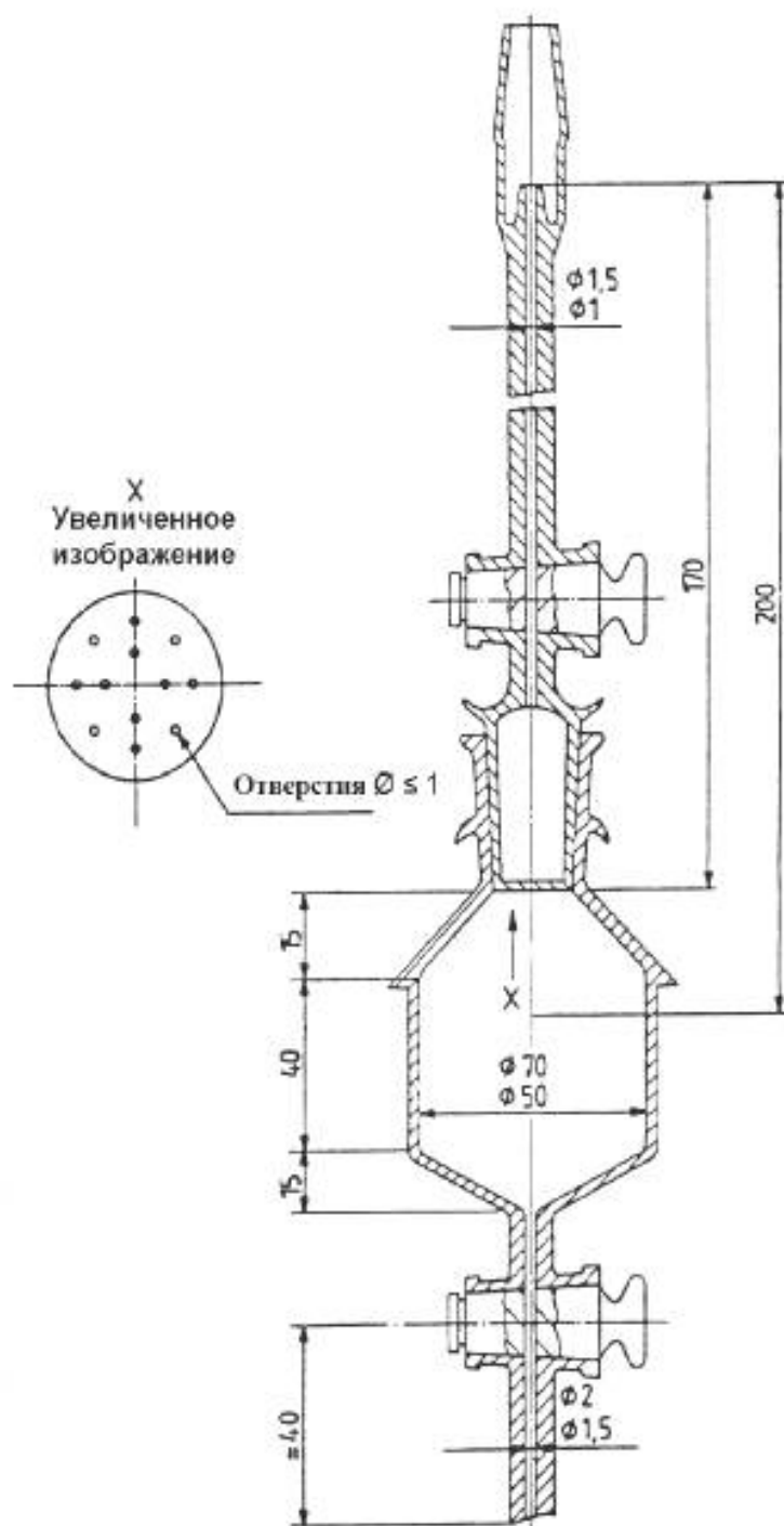
Рисунок 1 – Вакуумный пикнометр
