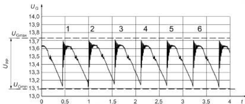
Рисунок 5 — Схематический вид колебаний напряжения ( p = 6 )
