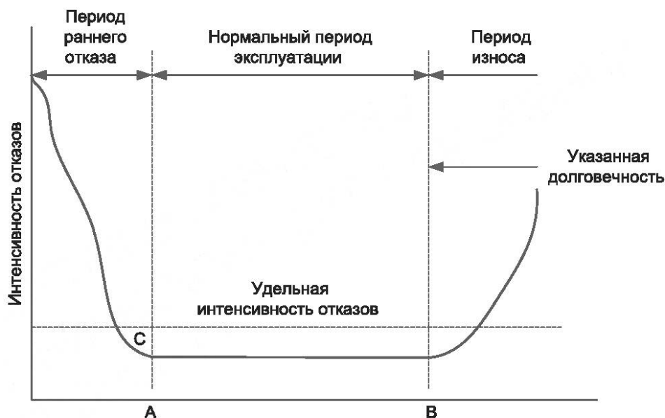
Рисунок С.1 — Кривая интенсивности отказов
