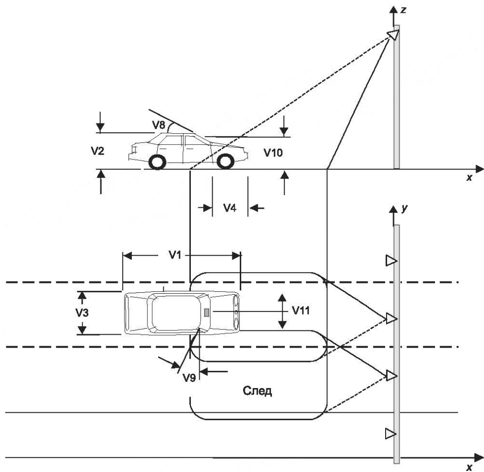
Рисунок 6 — Характеристики автомобиля
