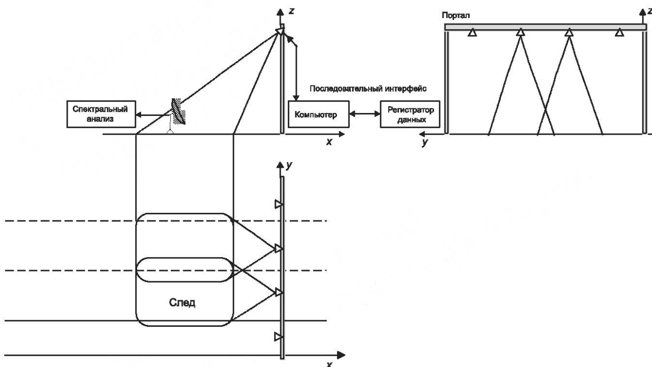
Рисунок F.1 — Тестовое оборудование для полевых испытаний
