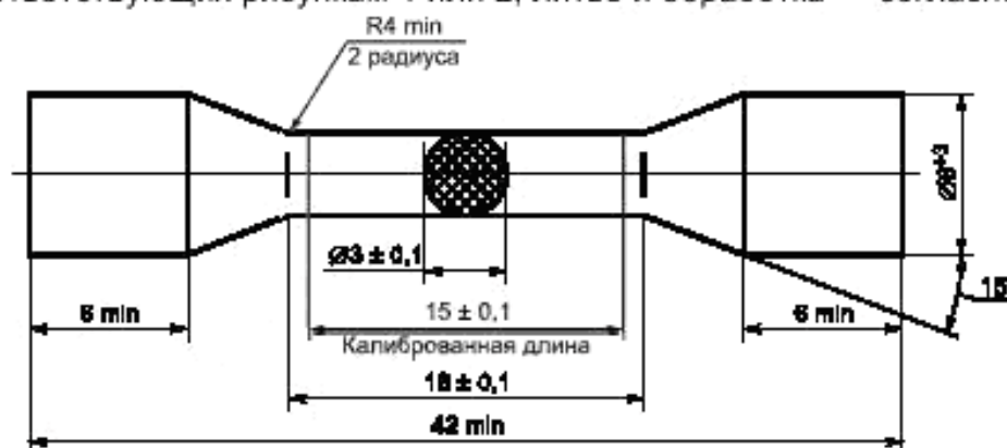
Рисунок 1 — Образец с короткой головкой
