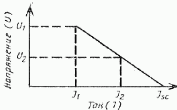
Рисунок 1 — Разрядная характеристика U=f(I)
