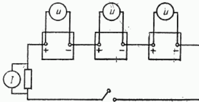
Рисунок 2 — Схема соединения
