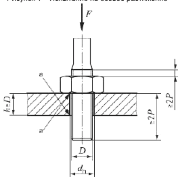
Рисунок 1 – Испытание на осевое растяжение
