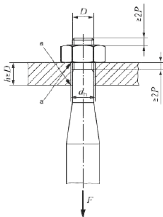
Рисунок 1 – Испытание на осевое растяжение
