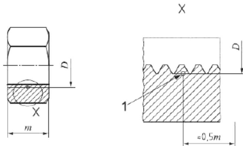
1 – Расположение точек измерения твердости
