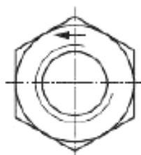
Рисунок 6 – Маркировка левой резьбы
