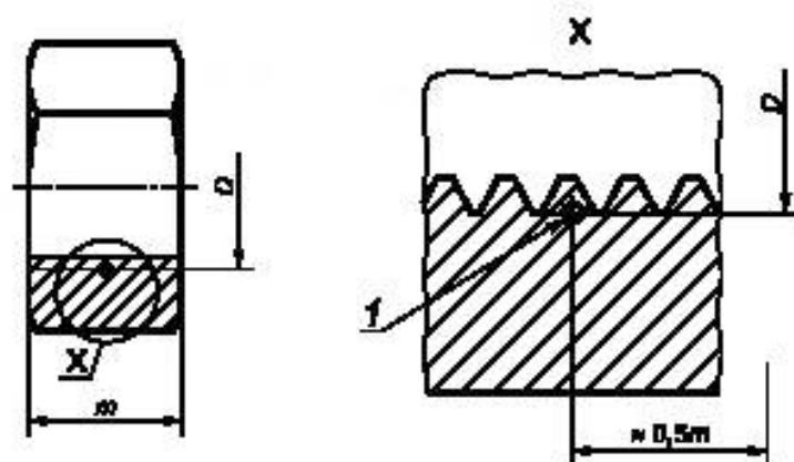
1 — Расположение точек измерения твердости
