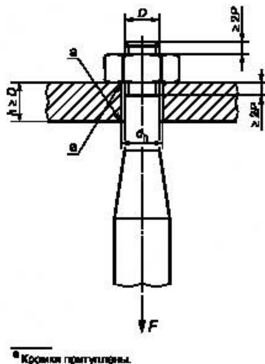
Рисунок 1 — Испытание на осевое растяжение
