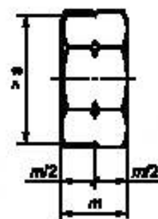
Рисунок 7 — Альтернативная маркировка левой резьбы
