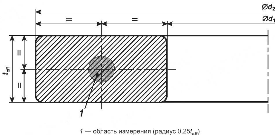
Рисунок 3 — Область измерения твердости
