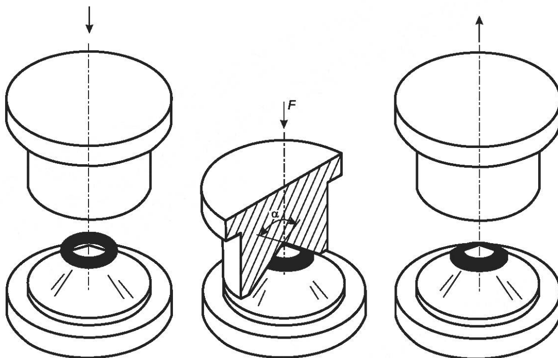
Рисунок А.1 — Пример испытательного устройства конической формы для шайб с концентрическими круглыми внутренним и внешним диаметрами
