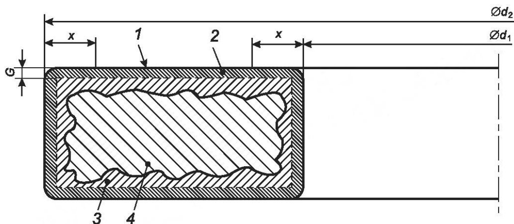
1 — опорная поверхность; 2 — полное обезуглероживание; 3 — частичное обезуглероживание; 4 — основной металл; x — зона, в которой не проводят испытание на обезуглероживание
