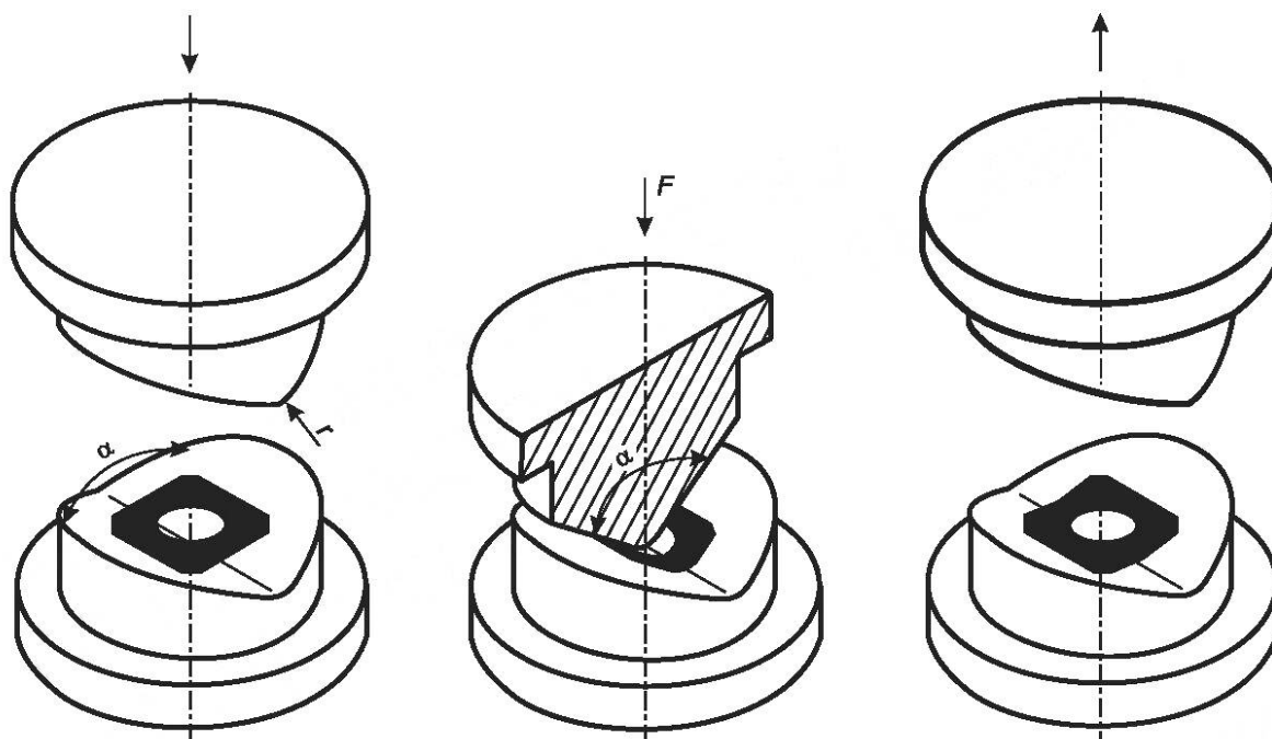
Рисунок А.2 — Пример испытательного устройства V-образной формы для шайб с другими формами
