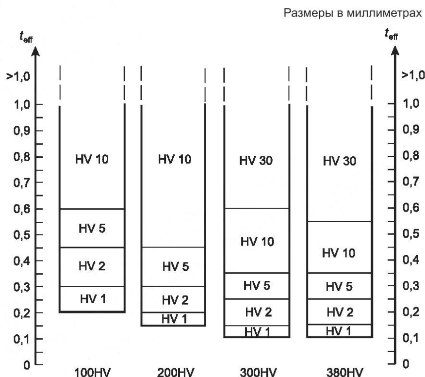
Рисунок 1 — Испытательное усилие для определения твердости по Виккерсу на опорной поверхности в зависимости от класса прочности и толщины шайбы
