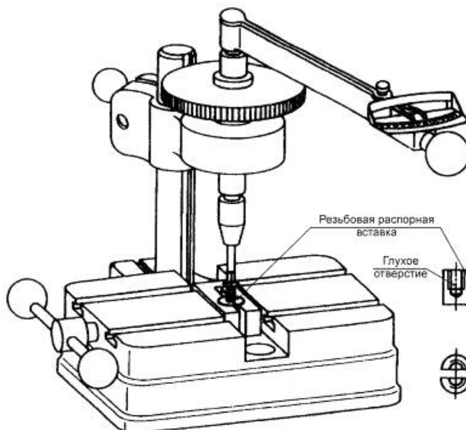
Рисунок 1 — Пример устройства для испытания на кручение
