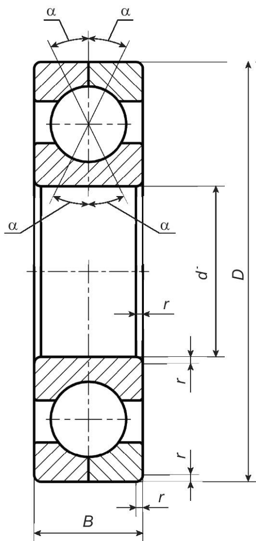
Рисунок 1 — Конструктивное исполнение 11
