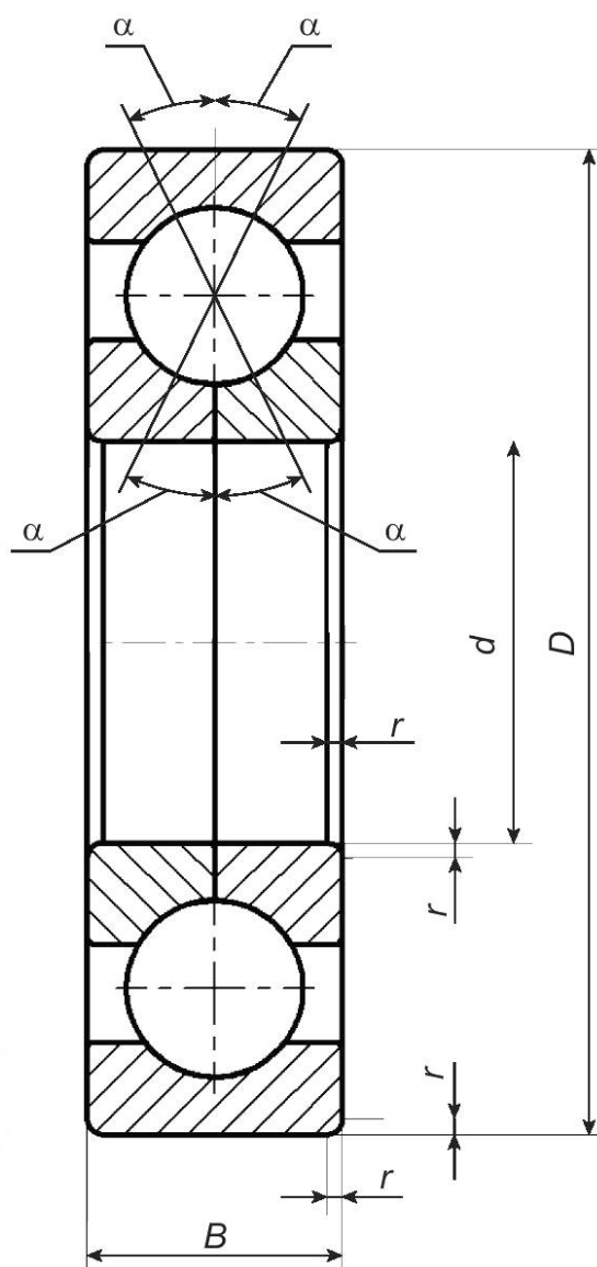
Рисунок 3 — Конструктивные исполнения 17, 59
