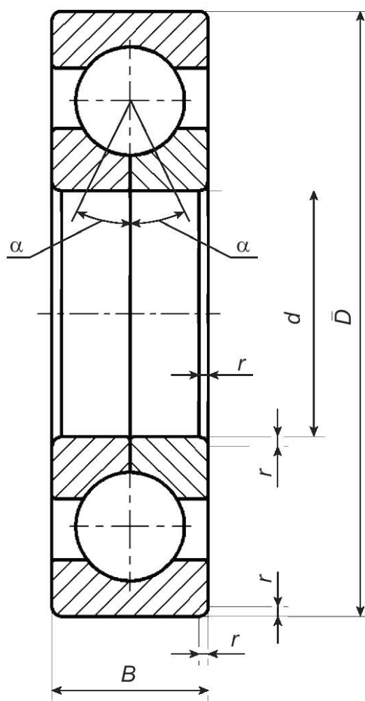
Рисунок 2 — Конструктивное исполнение 12
