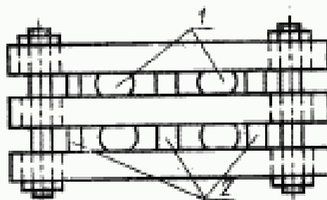
1—образцы, 2—ограничители
