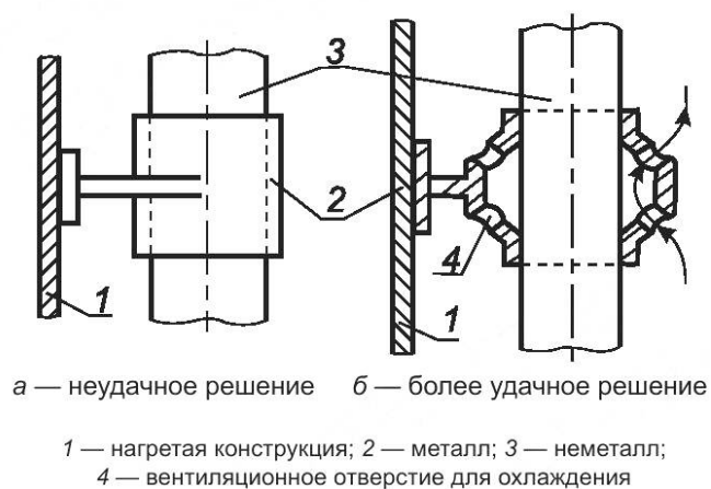
Рисунок Е.6 — Примеры геометрических форм кронштейнов пластиковых трубопроводов
