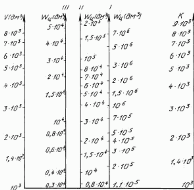
Расчет объема воды для противоточных схем промывок
