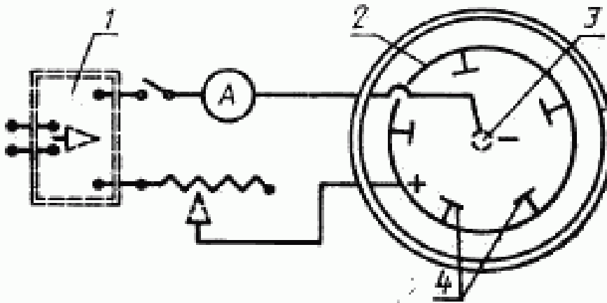
Схема установки катодной очистки пластины
