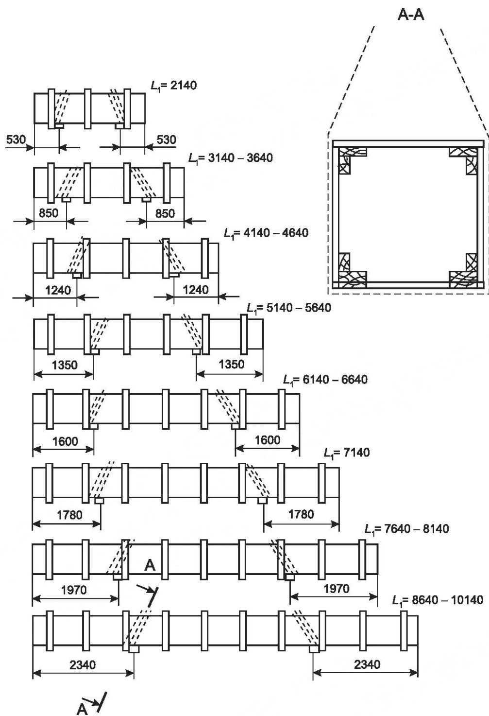
Рисунок Д.2 — Схемы строповки ящиков типов III и IV
