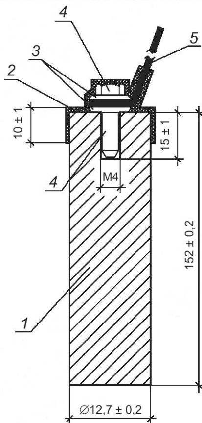
Рисунок 4 — Конструкция и рекомендуемые размеры образцов для измерения рабочего потенциала, фактической токоотдачи и КПД
