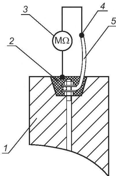
1 — рабочий элемент протектора; 2 — изоляция контактного узла; 3 — мегаомметр; 4 — места подключения контактов мегаомметра; 5 — соединительный кабель
