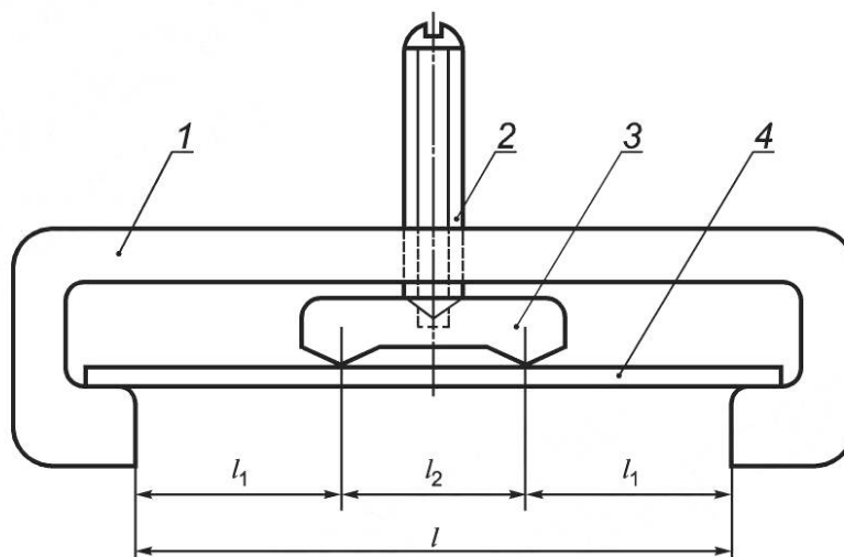
1 — скоба; 2 — шпилька; 3 — вкладыш; 4 — образец
