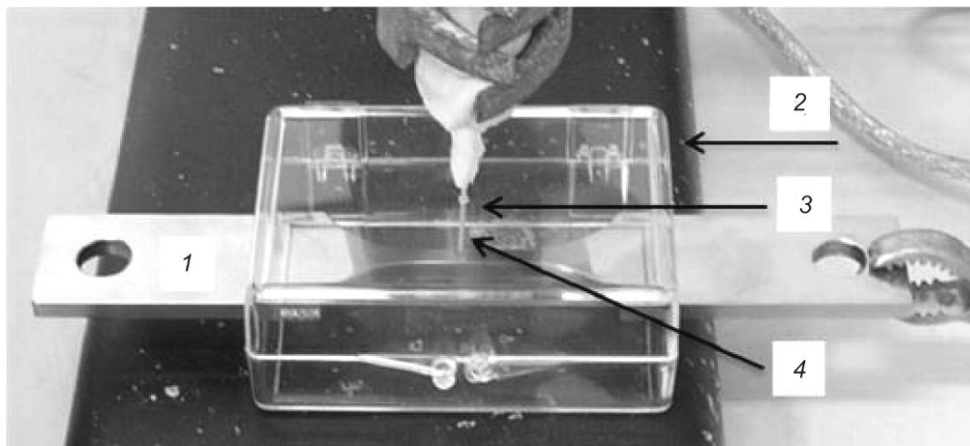
1 — испытуемый образец; 2 — ячейка для обработки каплями и минимизации их числа; 3 — электрод (платиновая проволока диаметром 0,1 мм); 4 — капилляр для подачи капель раствора (диаметром 0,5 мм)
