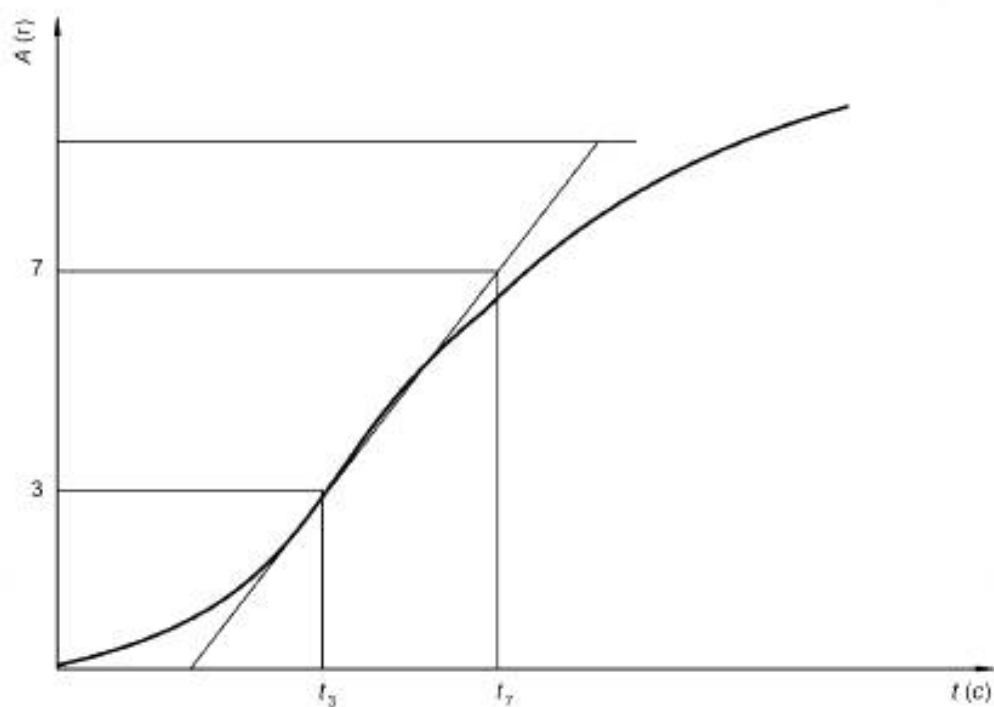
Рисунок А.2 — Калибровка пористой среды
