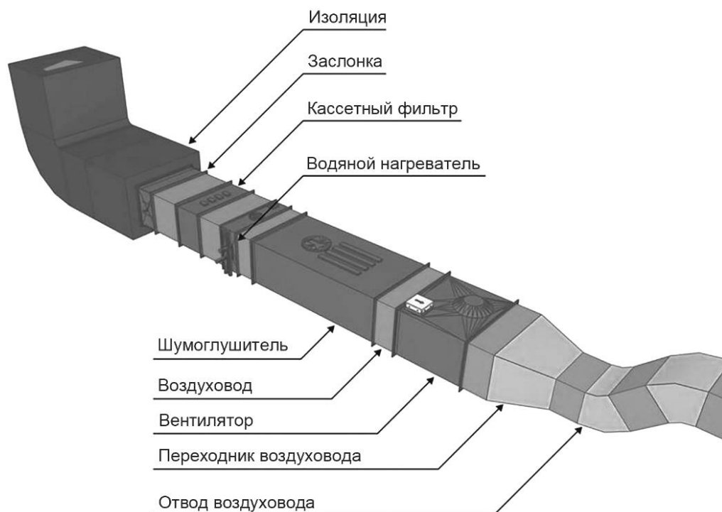
Рисунок 6 — Пример дисциплинарной ЦИМ вентиляции
