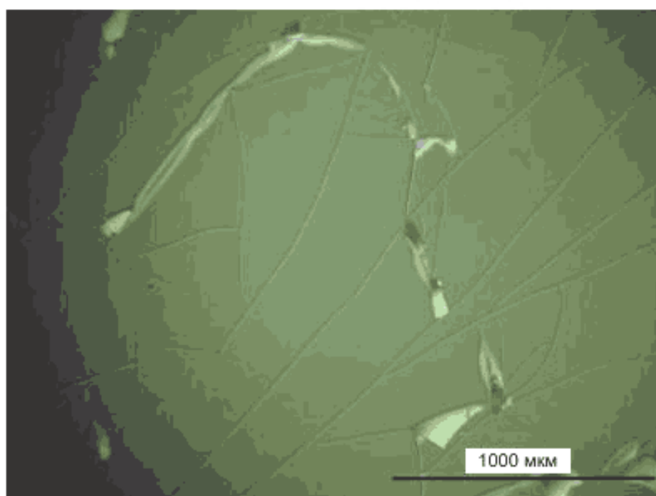
Рисунок А.8 – Трещина
