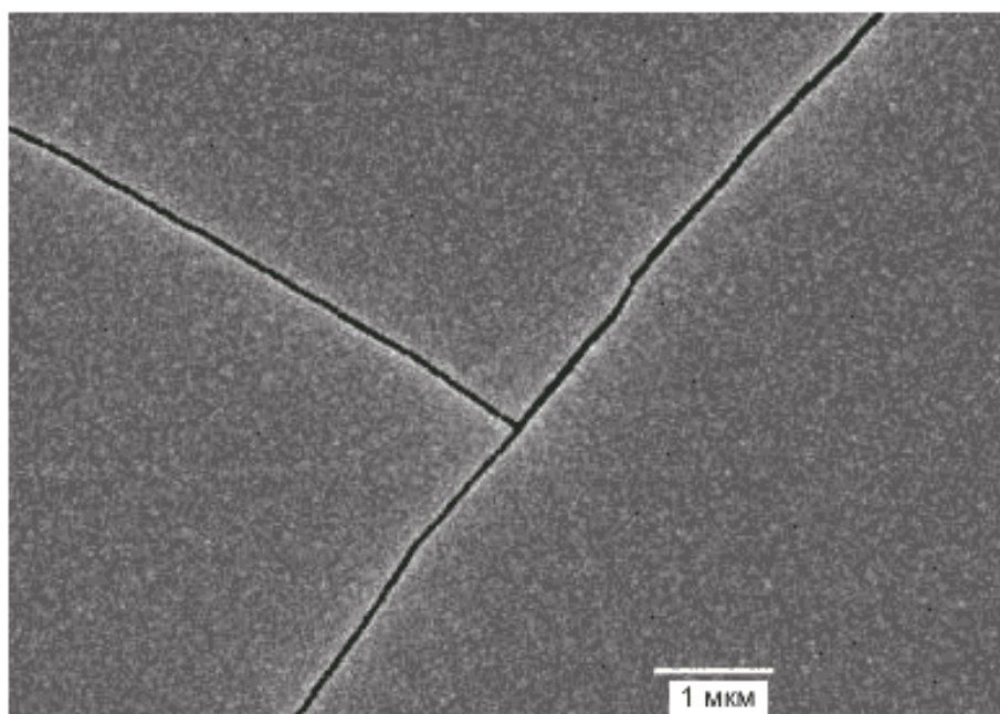
Рисунок А.9 – Волосные трещины
