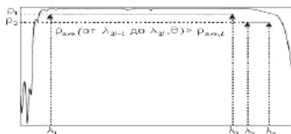
Рисунок 1 – Отражающая функция
