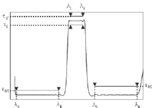
Рисунок 5 – Пропускающая функция
