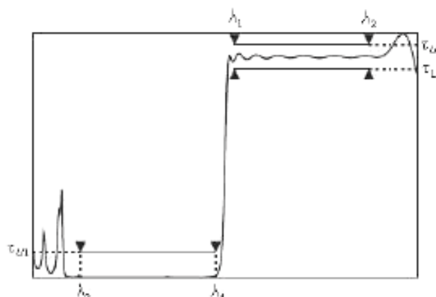
Рисунок 7 – Избирательная (комбинирующая) функция в длинноволновой области спектра
