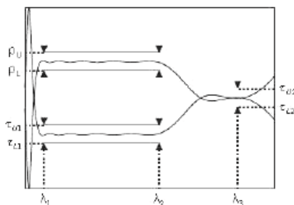
Рисунок 3 – Светоделительная функция
