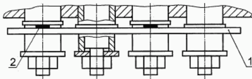
1 — поверочная линейка; 2 — щуп
