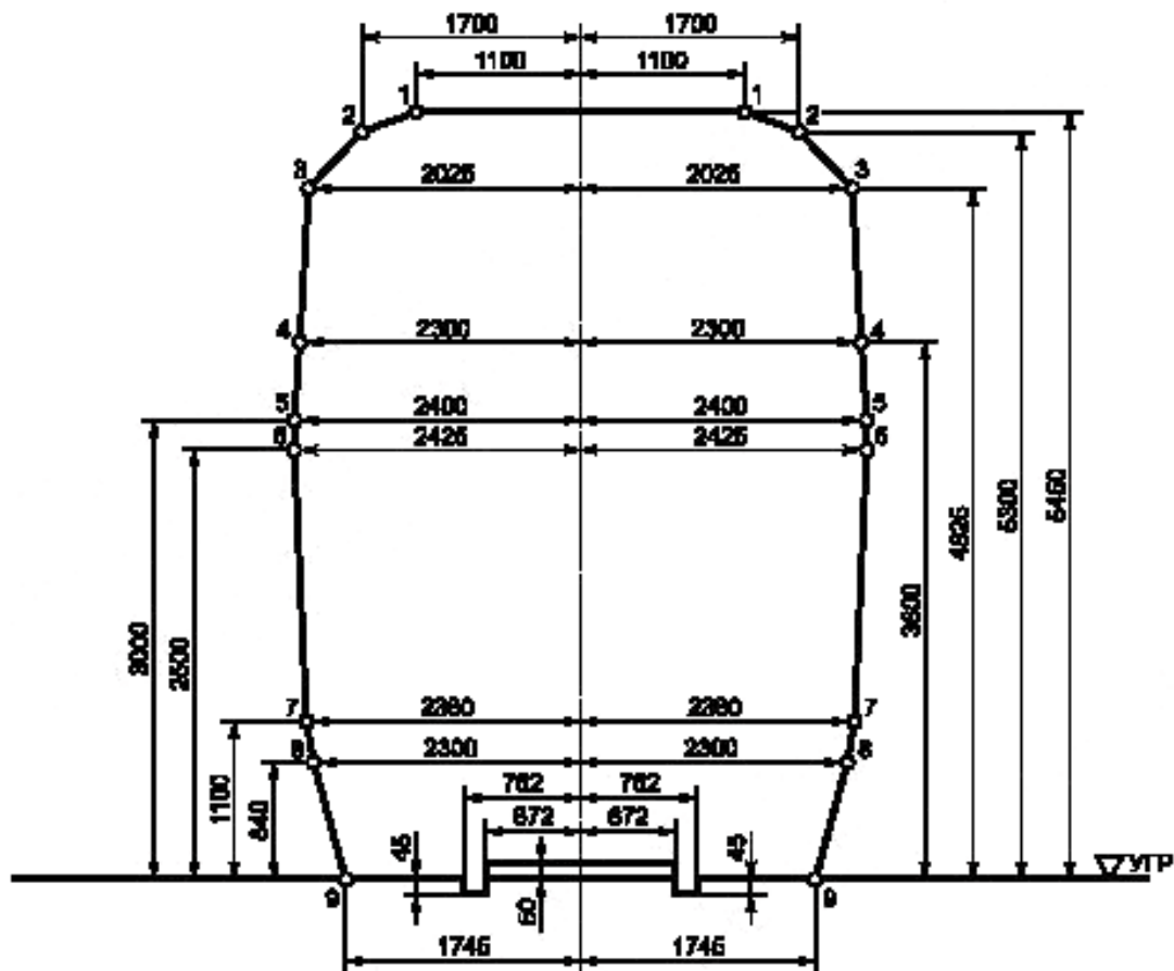
Рисунок В.3 — Минимальное внутреннее очертание переустраиваемых существующих сооружений (для незлектрифицированных линий)
