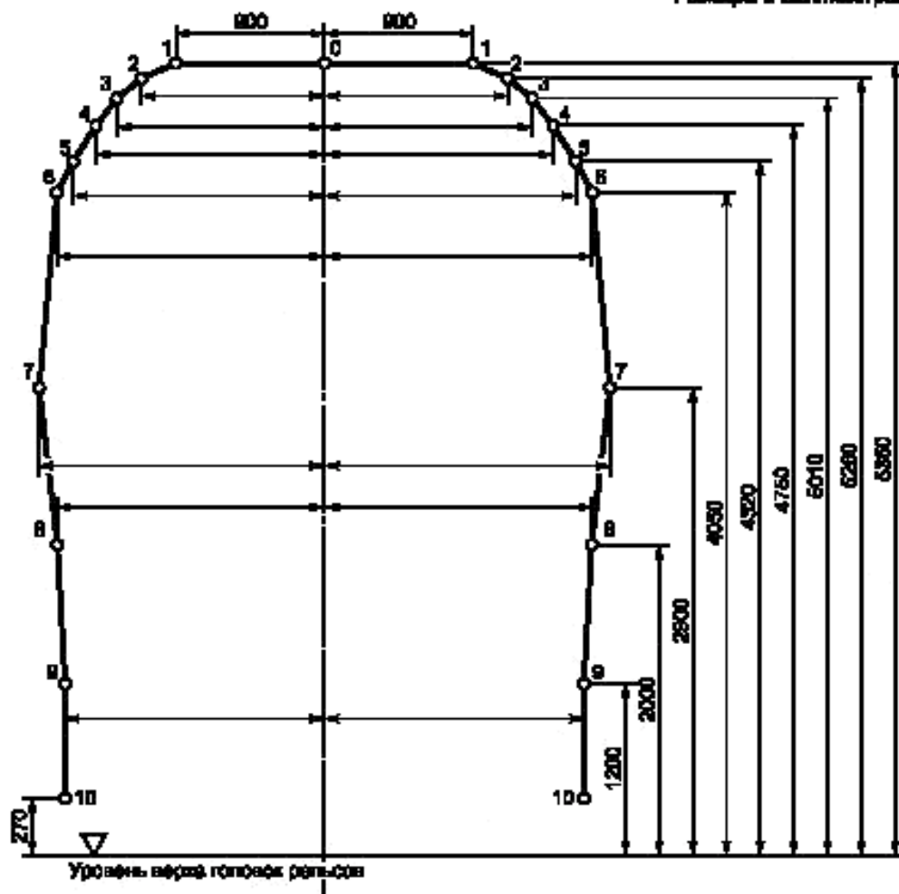
Рисунок Г.2 — Контрольное очертание сооружений Ц для пропуска подвижного состава габарита T_{\text{ч}} при скорости движения более 40 км/ч
