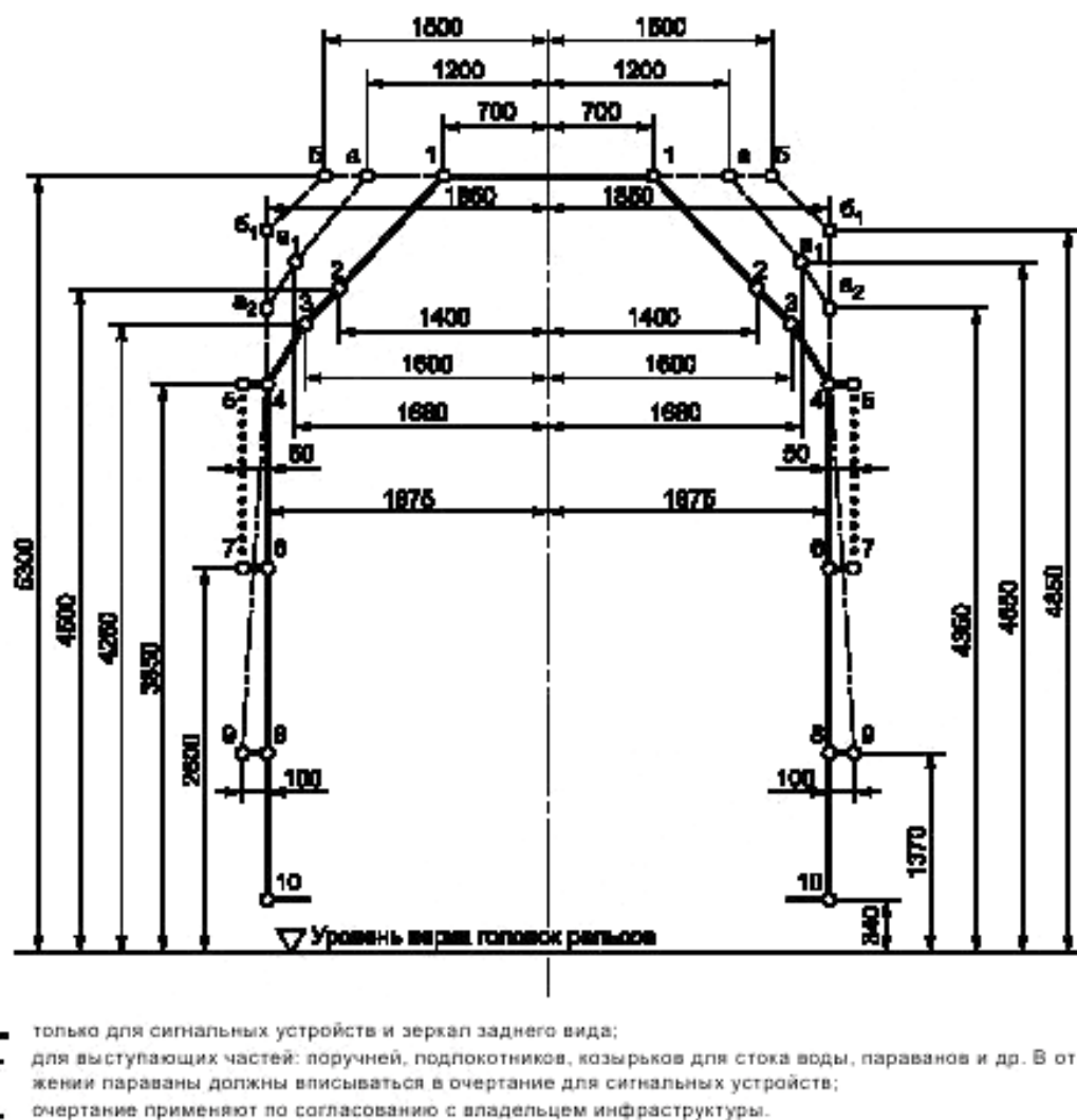
Рисунок 1 — Статический габарит Т
