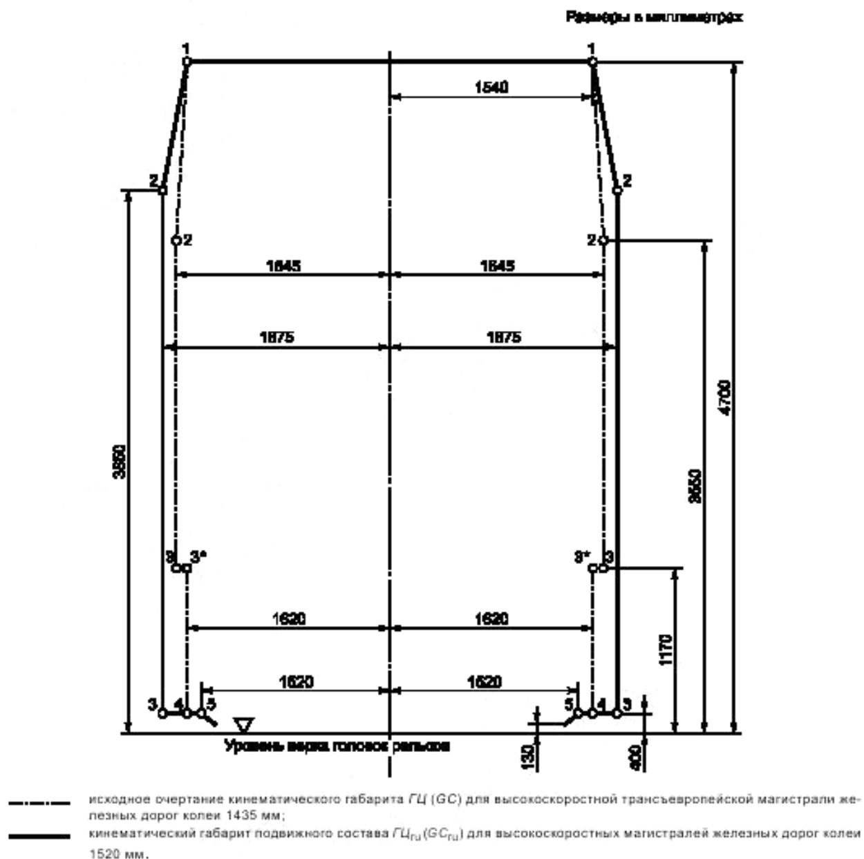
Рисунок 9 — Габарит подвижного состава ГЦ ( GC ) и гармонизированный с ним габарит ГЦ_{гн} ( GC_{гн} )
