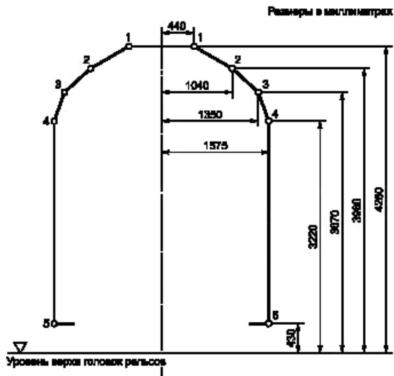
Рисунок 13 — Статический габарит 03-ВМ 1
