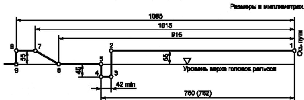
Рисунок 27 — Нижнее очертание габаритов S и S_n для двойных перекрестных стрелочных переводов, планов контроля нижнего габарита, устройств контроля схода подвижного состава
