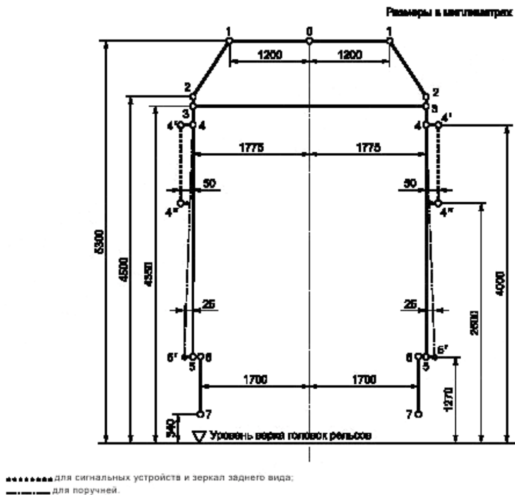
Рисунок 3 — Статический габарит T_{пр}
