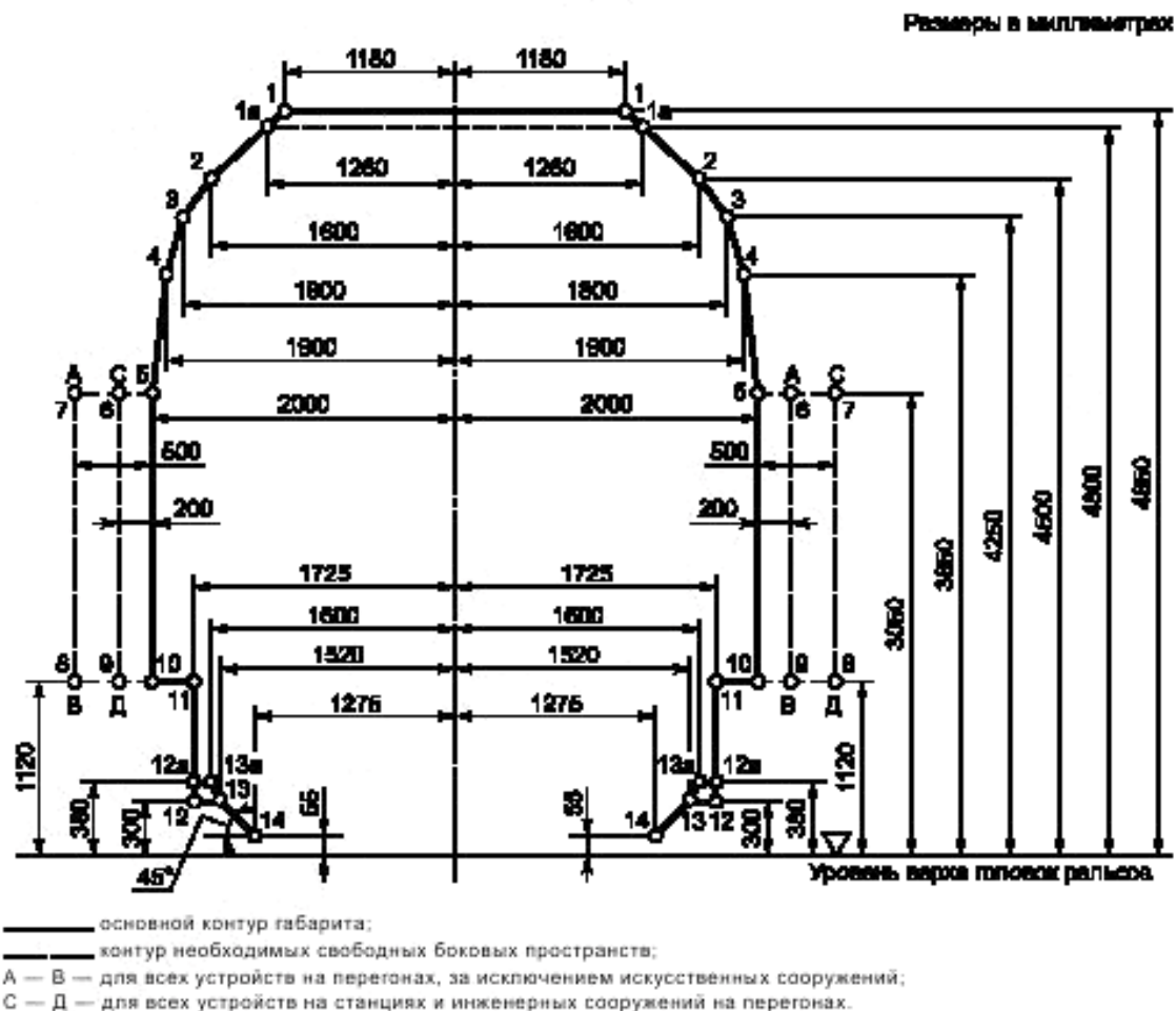
Рисунок Б.1 — Верхнее очертание габарита 1-СМ
