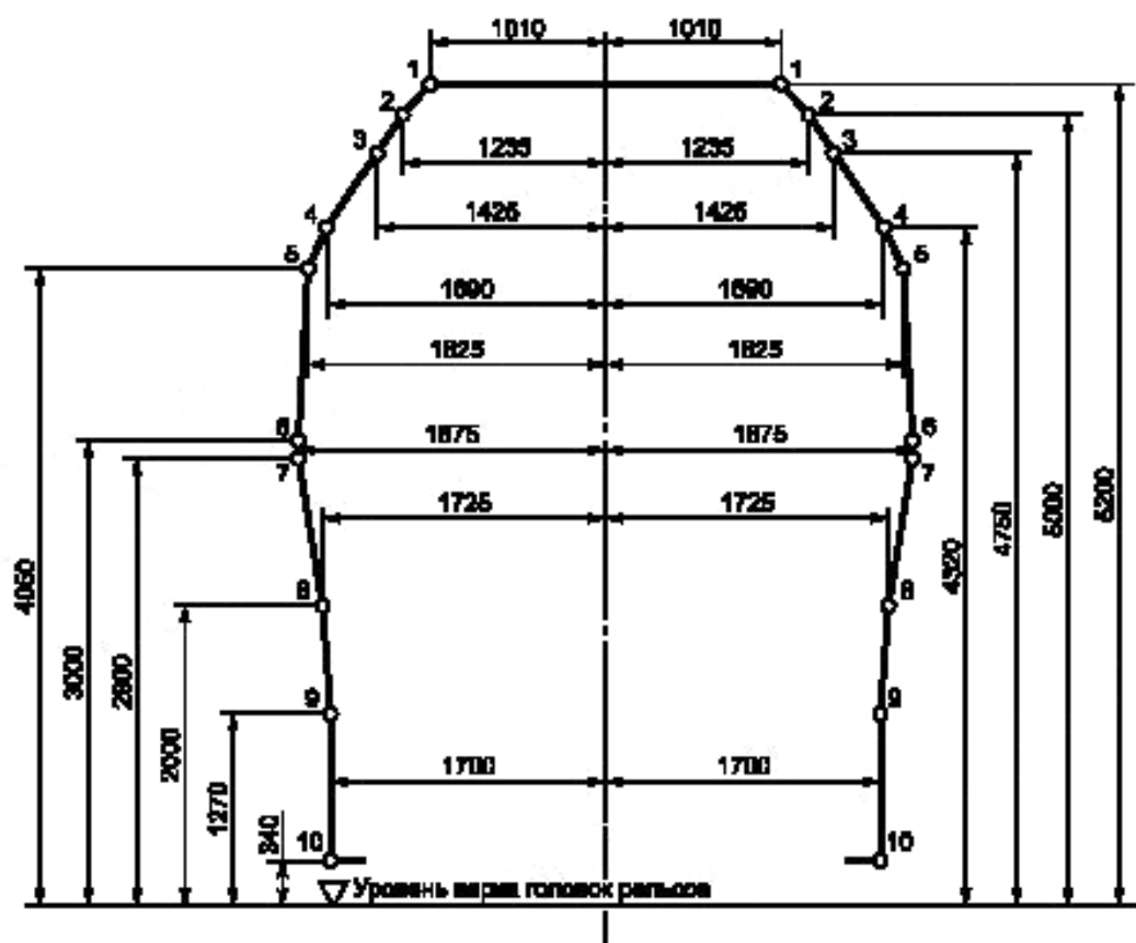
Рисунок 2 — Статический габарит T_{\text{ц}}
