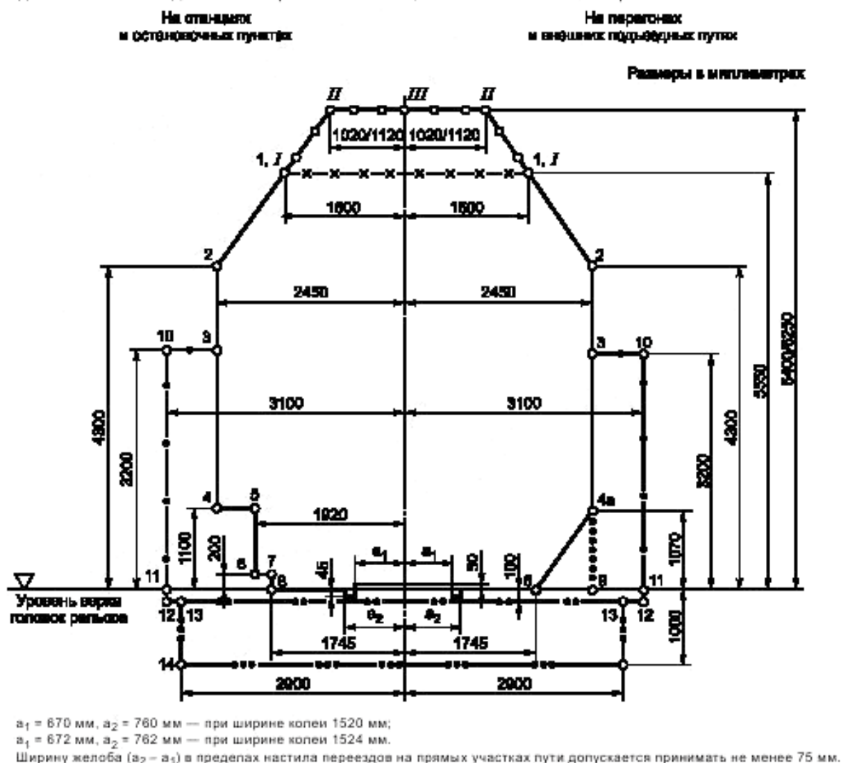
Рисунок 24 — Габарит С
