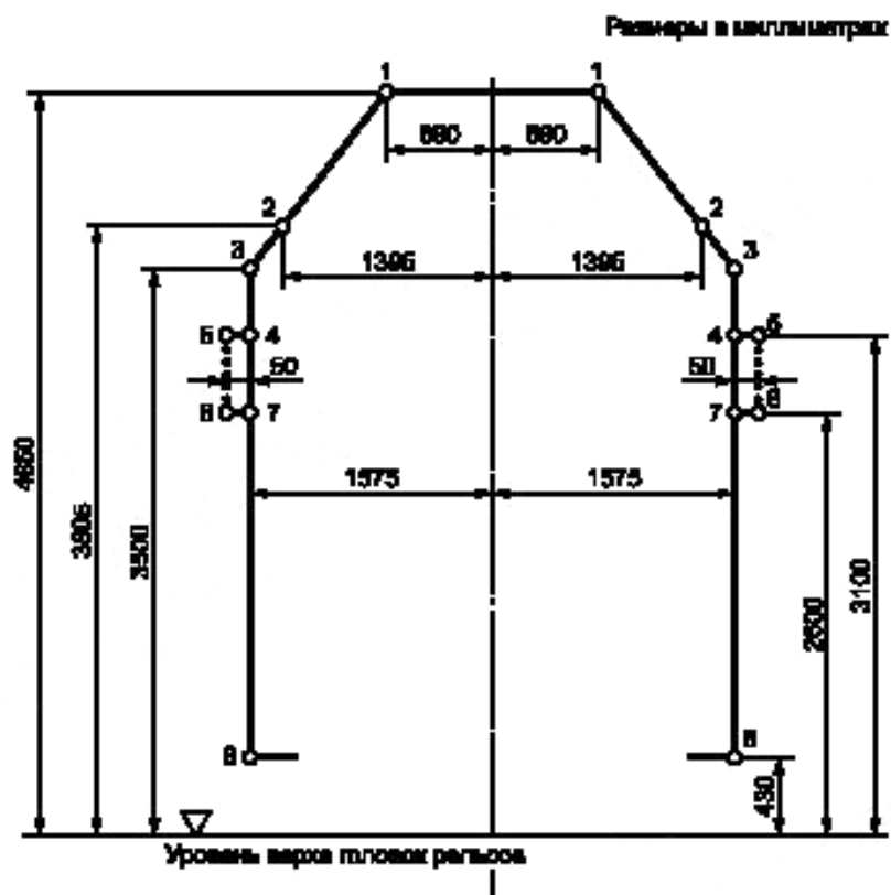
Рисунок 12 — Статический габарит 02-ВМ
