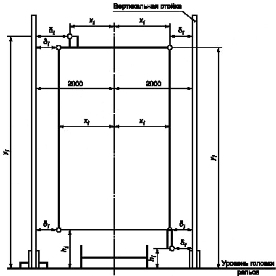
Рисунок И.1 — Схема измерения габаритных размеров
