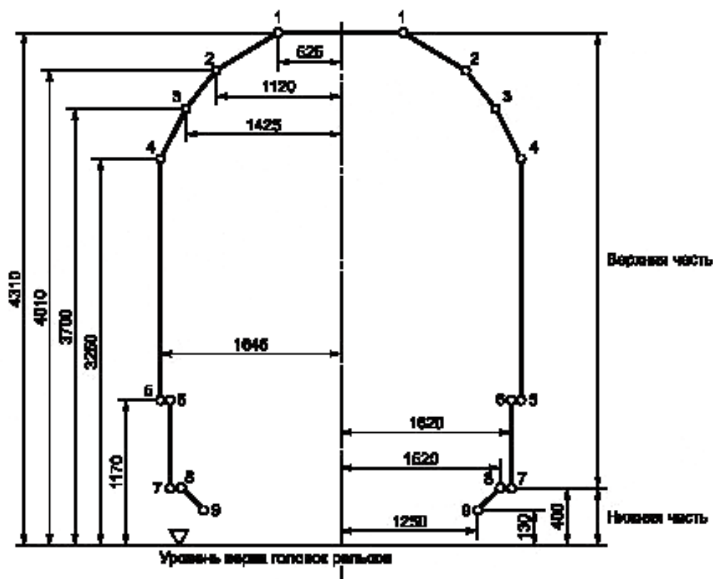
Рисунок 14 — Кинематический габарит 03-ВМ.
