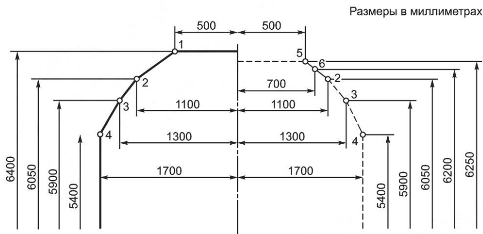
Рисунок Д.1 — Минимальное очертание верхней части сооружений при напряжении в контактной сети 25 кВ
