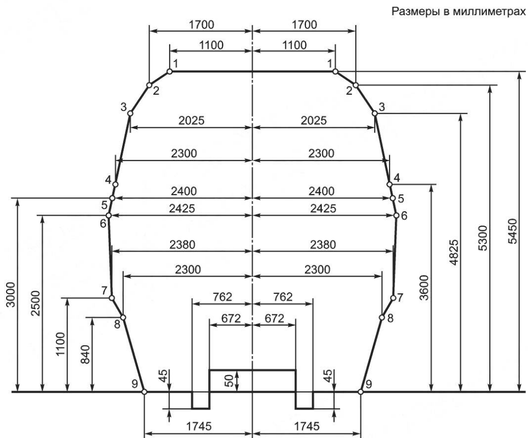
Рисунок Д.3 — Минимальное внутреннее очертание переустраиваемых существующих сооружений (для не электрифицированных линий)
