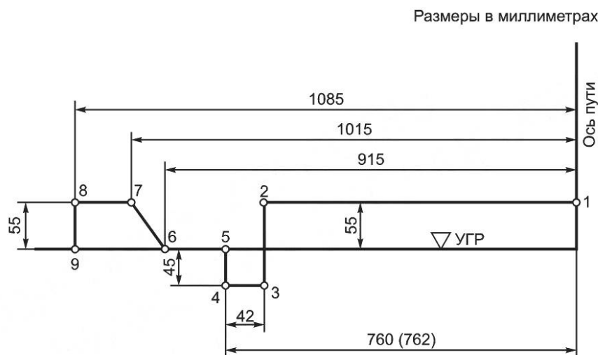
Рисунок 27 — Нижнее очертание габаритов С и С п для двойных перекрестных стрелочных переводов, планок контроля нижнего габарита, устройств контроля схода подвижного состава
