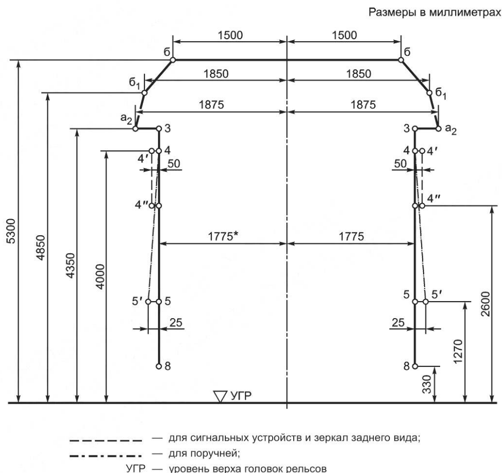
Рисунок Г.1 — Верхнее очертание статического габарита T_d для двухэтажных пассажирских вагонов локомотивной тяги и моторвагонного подвижного состава
