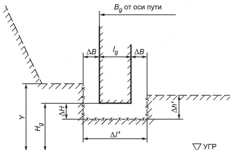
Рисунок Л.4 — Схема определения вертикального выреза для негабаритной детали
