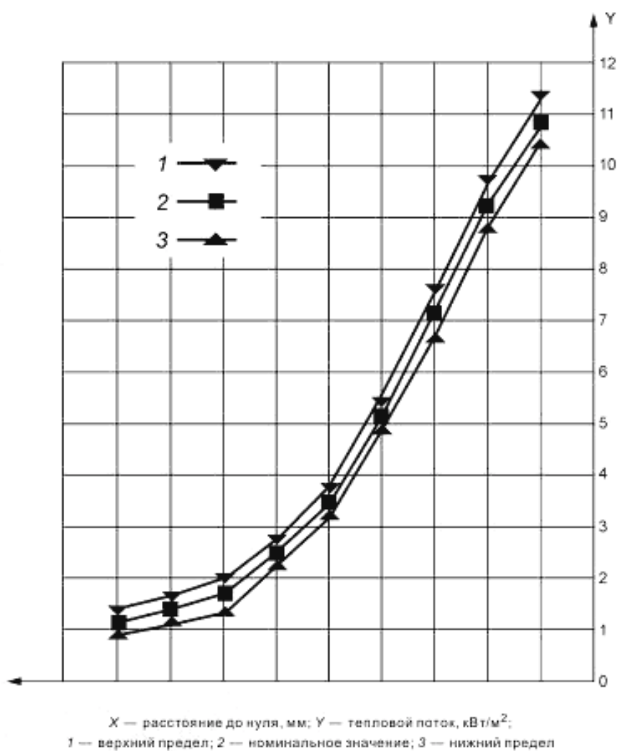
Рисунок 9 — График распределения плотности теплового потока
