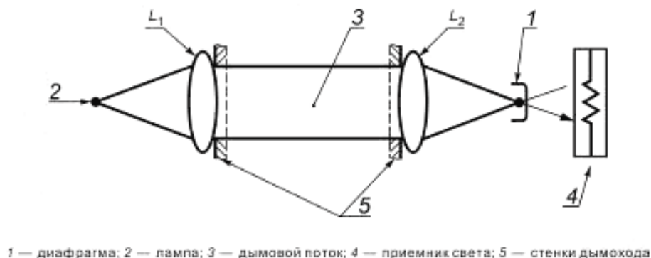
Рисунок А.1 — Оптическая система
