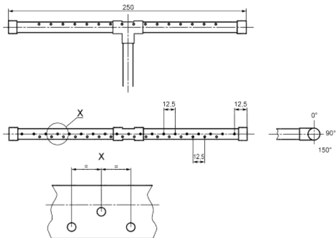
Рисунок 7 — Горелка
