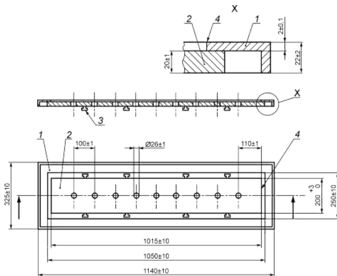
Рисунок 6 — Держатель образца с калибровочным образцом
