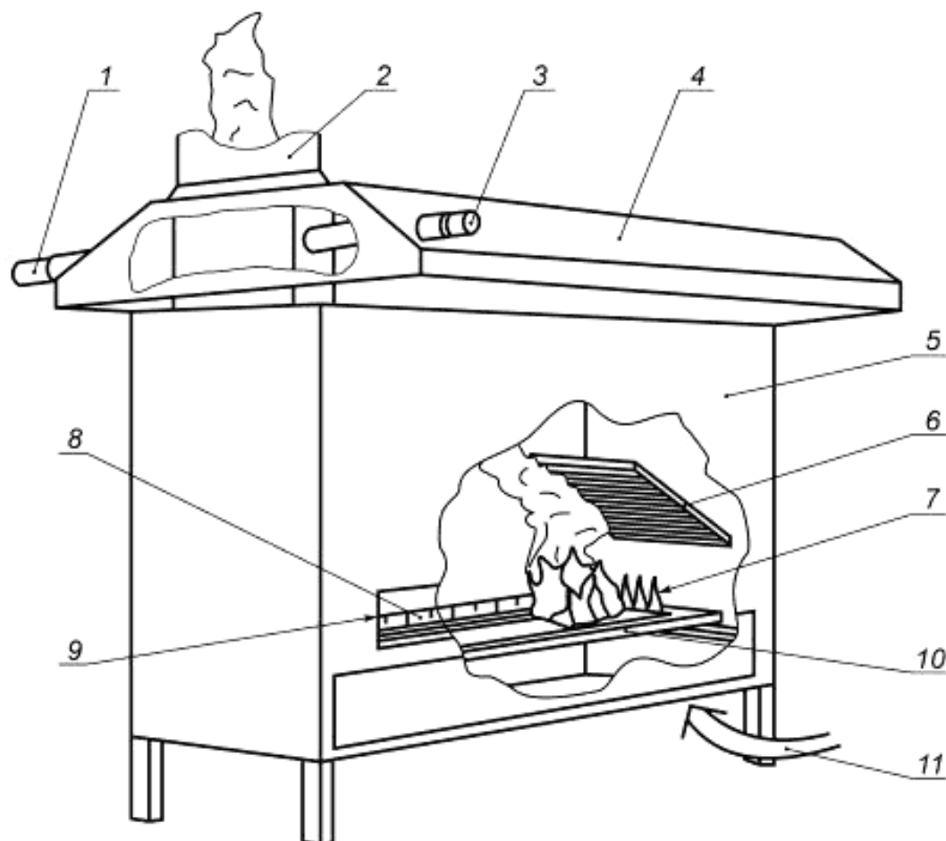
1 — лампа; 2 — вытяжка; 3 — приемник света; 4 — вытяжной зонтик; 5 — испытательная камера; 6 — поджигаемая газом излучающая панель; 7 — пилотное пламя от линии горелок; 8 — линейка; 9 — окно наблюдения; 10 — держатель образца с испытательным образцом и со скользящей платформой; 11 — доступ воздуха вокруг испытательного образца внизу камеры
