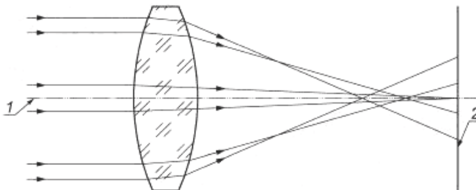
1 – оптическая ось; 2 – параксиальный фокус
