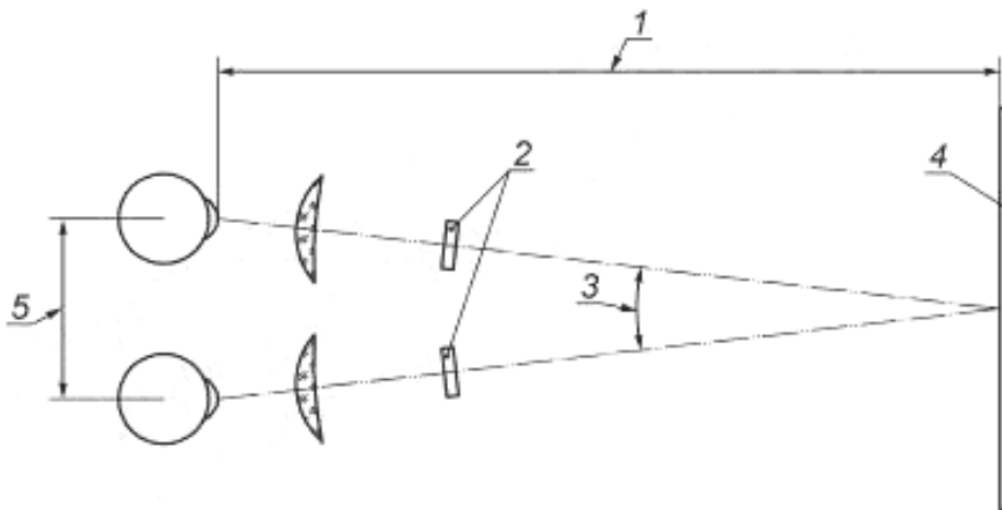
Рисунок 12 – Точка сходимости
