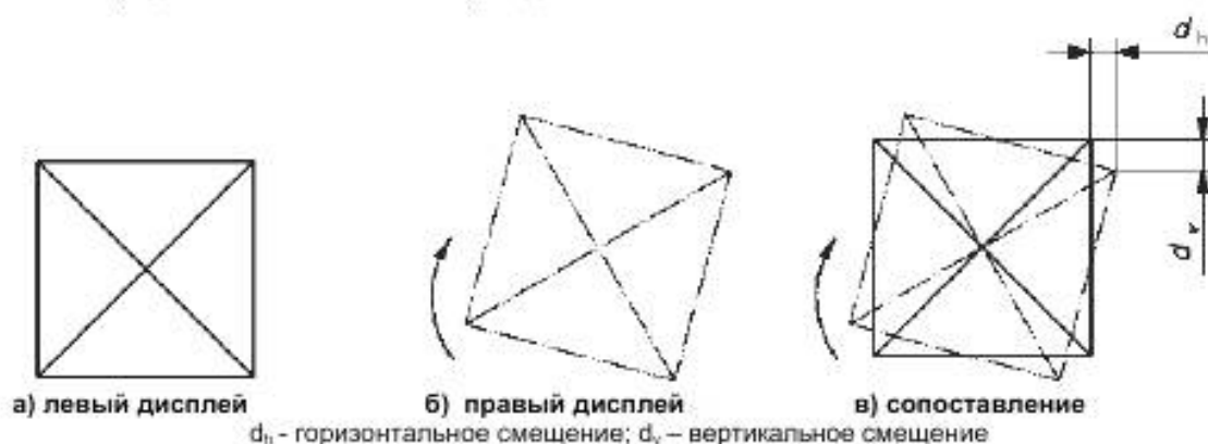
Рисунок Е.4 - Межглазная разность вращения
