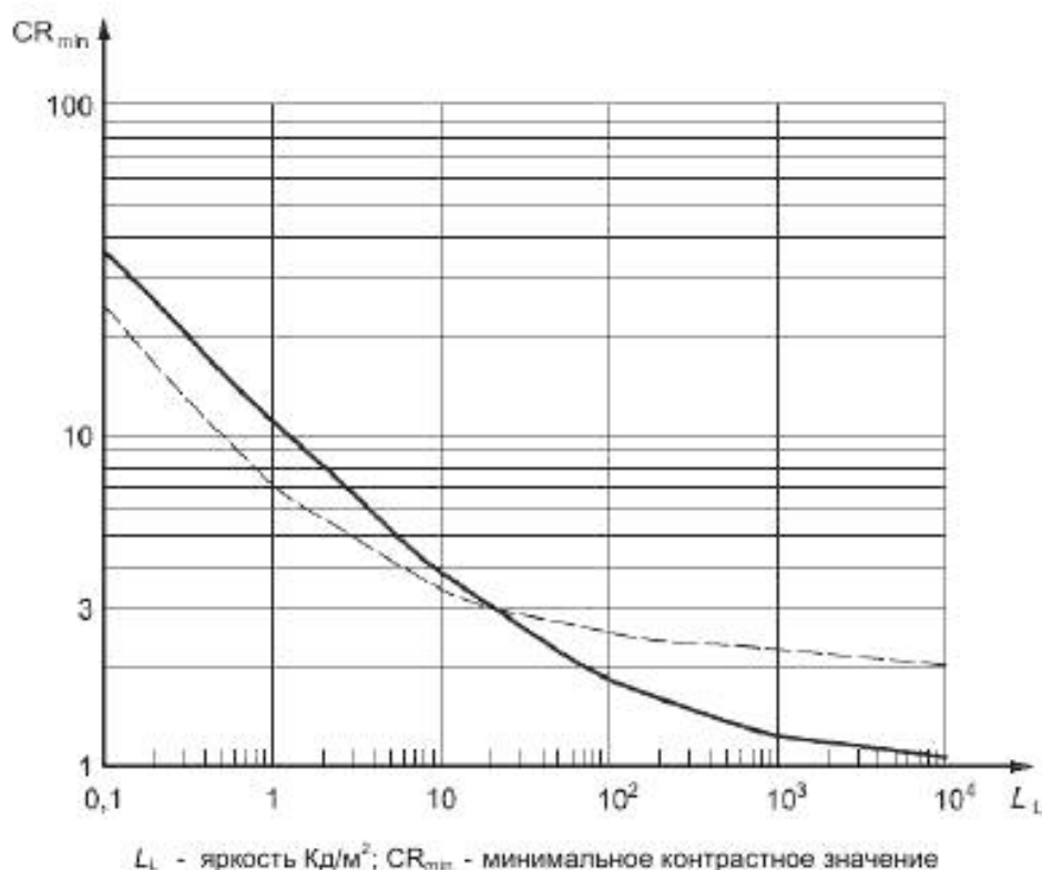
Рисунок D.3- Требуемый минимальный контраст дисплеев
