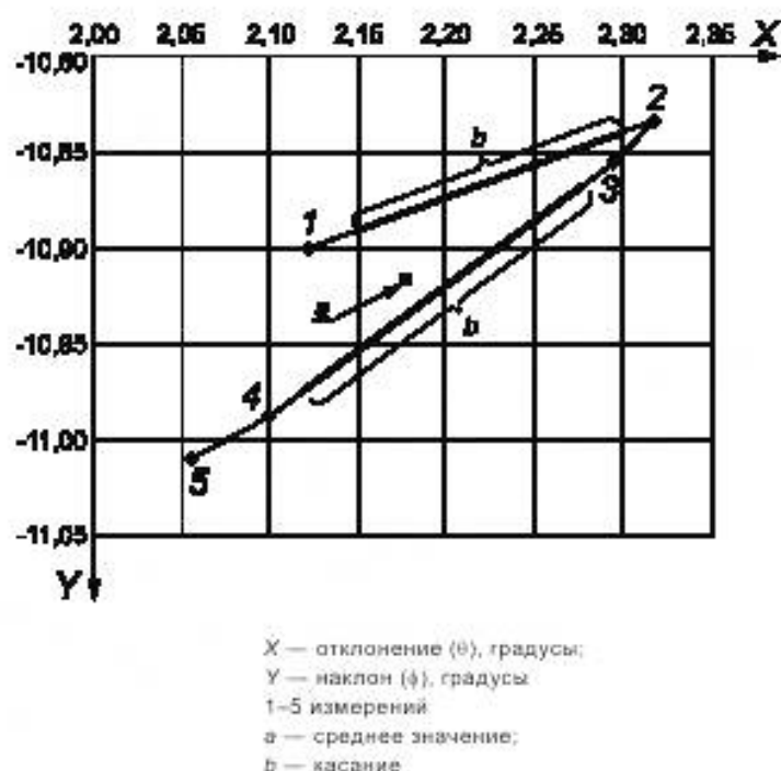
Рисунок 71 — «Неудачный» набор данных измерения
