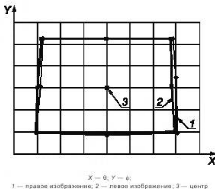
Рисунок 73 — Графики искажения при совмещении левого и правого изображений
