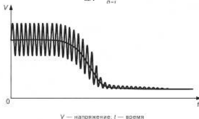
Рисунок 53 — Кривая переходной характеристики (SRF) с периодической пульсацией
