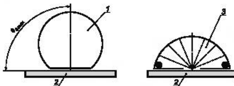
1 — фотометрический шар; 2 — ИО; 3 — диффузная полусфера
