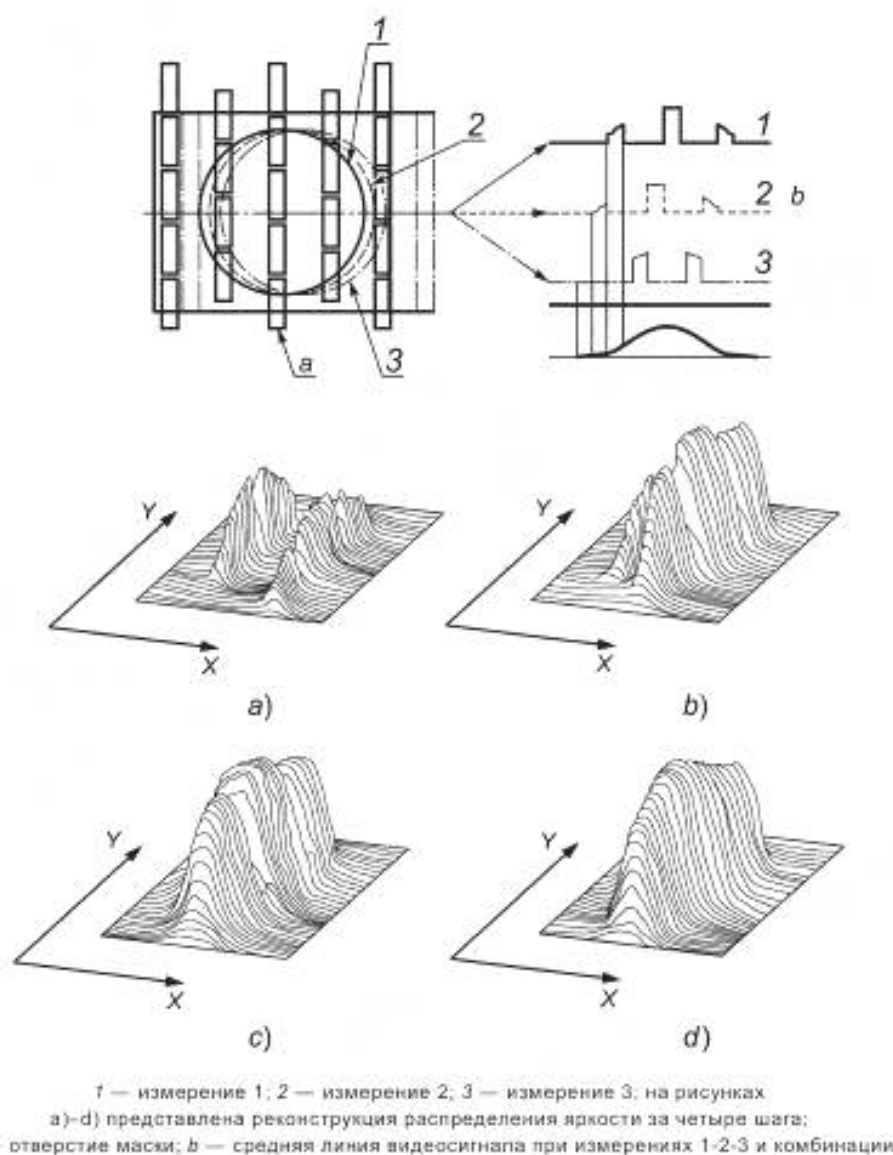
Рисунок F.1 — Реконструкция распределения яркости
