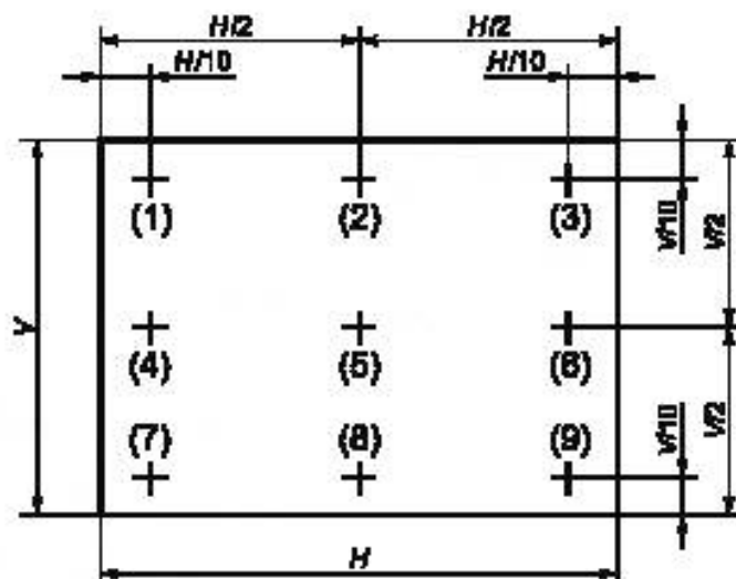
Рисунок 37 — Альтернативное расположение девяти точек измерения (VESA)
