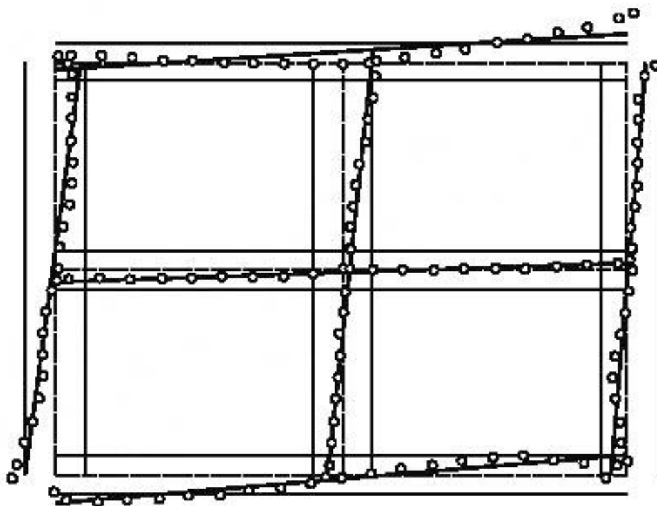
Рисунок 66 — Погрешности волнистости (увеличение в 50 раз для ясности)
