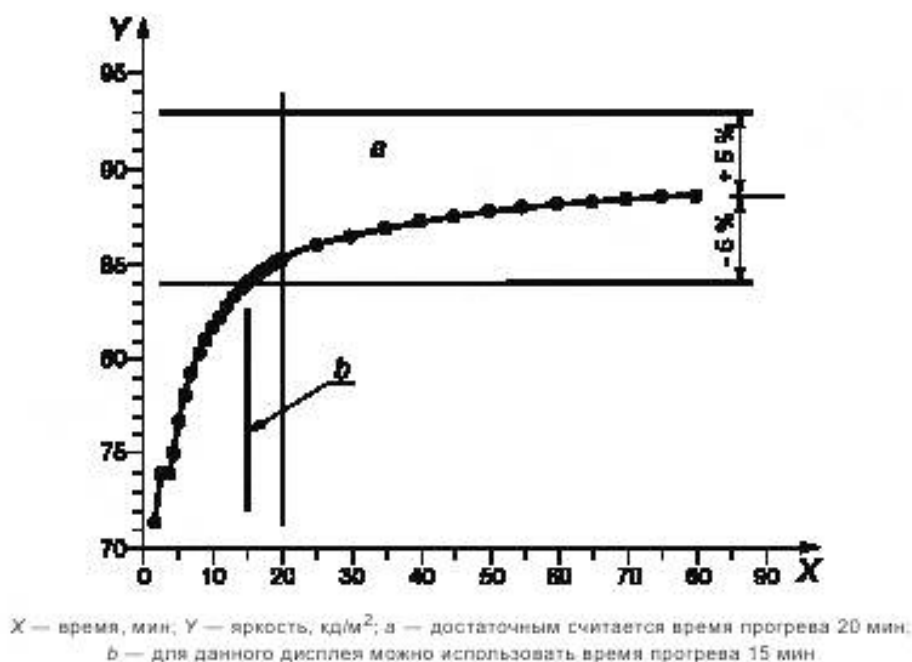
Рисунок 56 — Время прогрева
