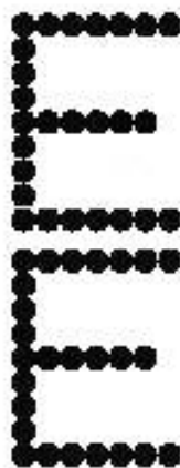
Рисунок 11 — Межстрочный интервал
