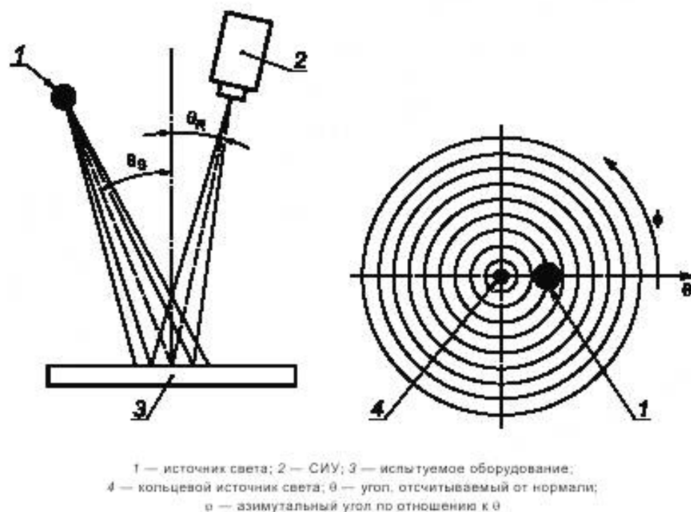
Рисунок 39 — Направленное освещение [18]
