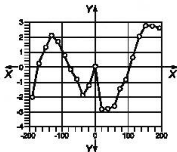
а) Линейность по горизонтали
