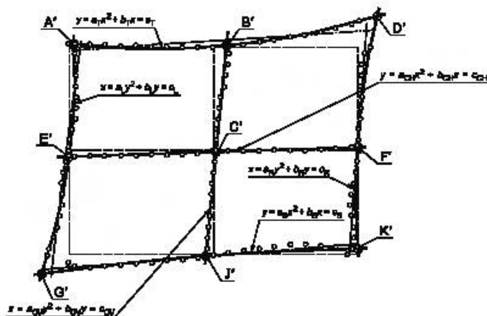
Рисунок 69 — Анализ подушкообразного искажения
