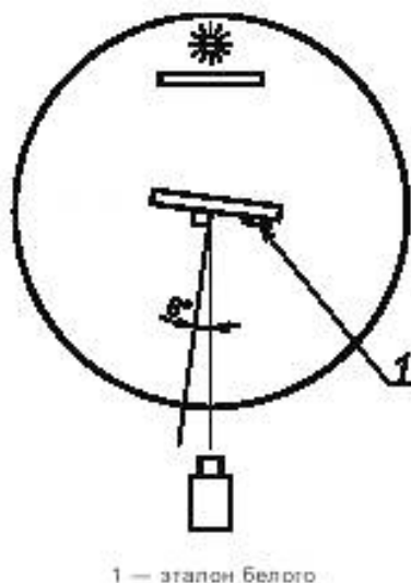
Рисунок 50 — Конфигурация диффузной сферы
