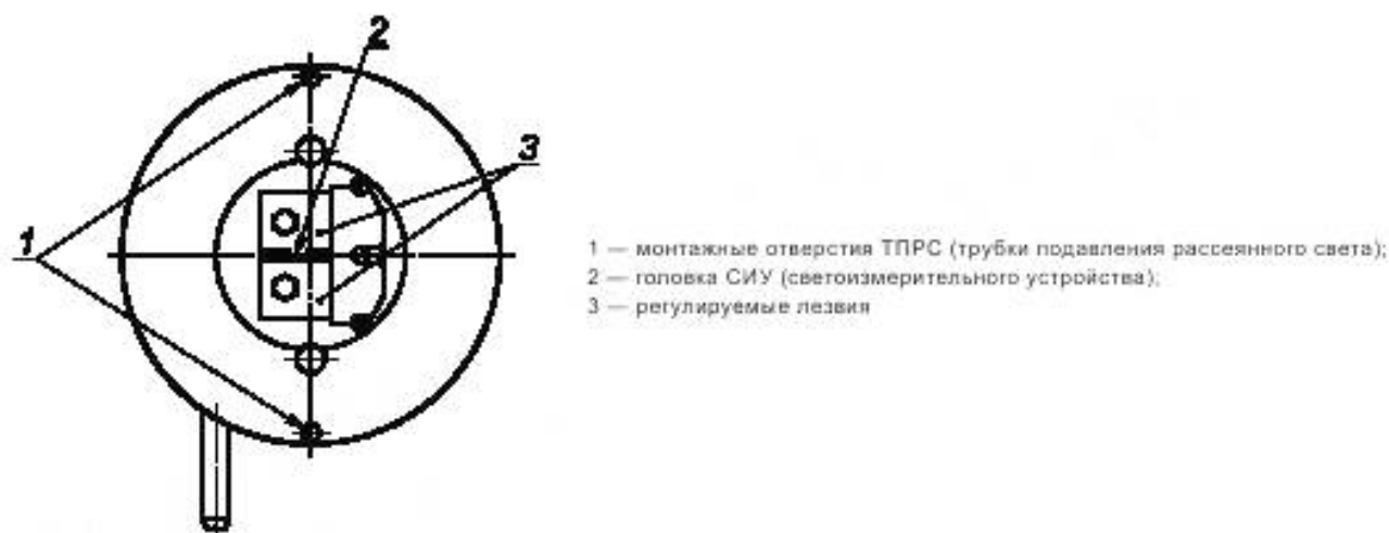
Рисунок 3 — Щелевая оправка для измерителя освещенности
