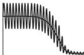
Рисунок 51— Кривая переходной характеристики с периодической пульсацией
