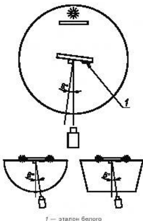
Рисунок 5 — Сферическая и полусферическая окружающая оболочка
