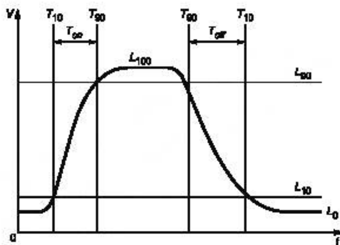
Рисунок 52 — Пример быстродействий
