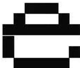
Рисунок 15 — Изображение «е»
