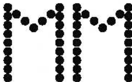
Рисунок 9 — Межзнаковый интервал
