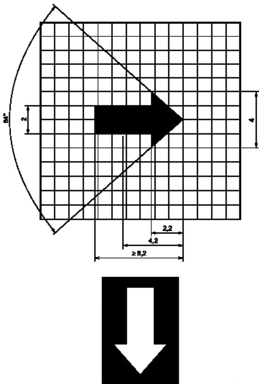
Рисунок D.22 — Стрелка, обозначающая давление или силу
