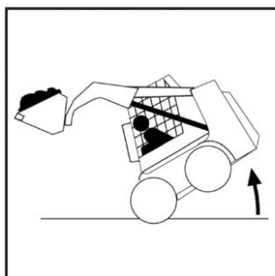
Рисунок А.42 — Опрокидывание машины. Перегруз. Минипогрузчик
