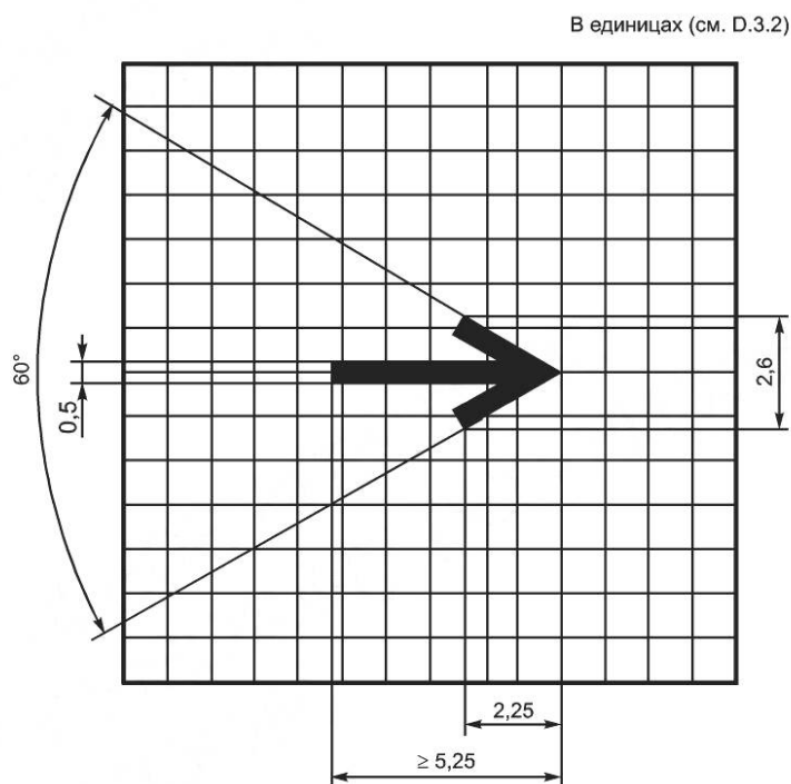
Рисунок D.20 — Стрелка, обозначающая направление движения машины в целом
