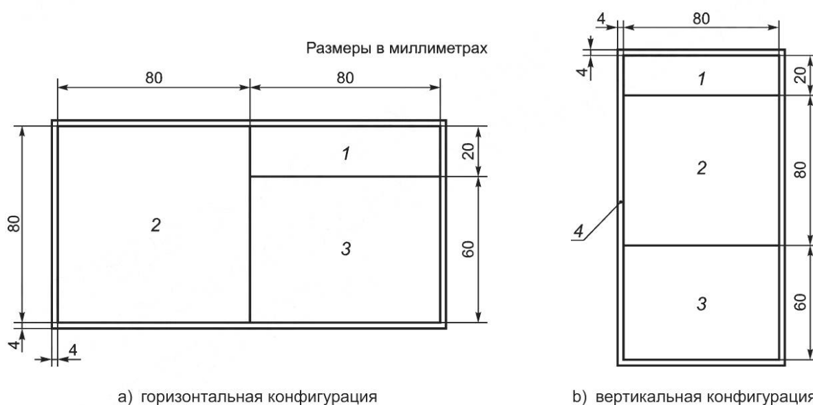
Рисунок 12 — Рекомендуемые размеры. Двухпанельный формат
