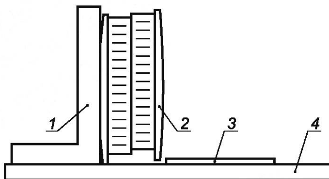
1 — угольник; 2 — блок; 3 — щуп; 4 — поверочная плита
