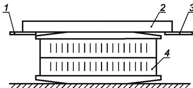
1 — 1-й щуп; 2 — поверочная линейка; 3 — 2-й щуп; 4 — блок
