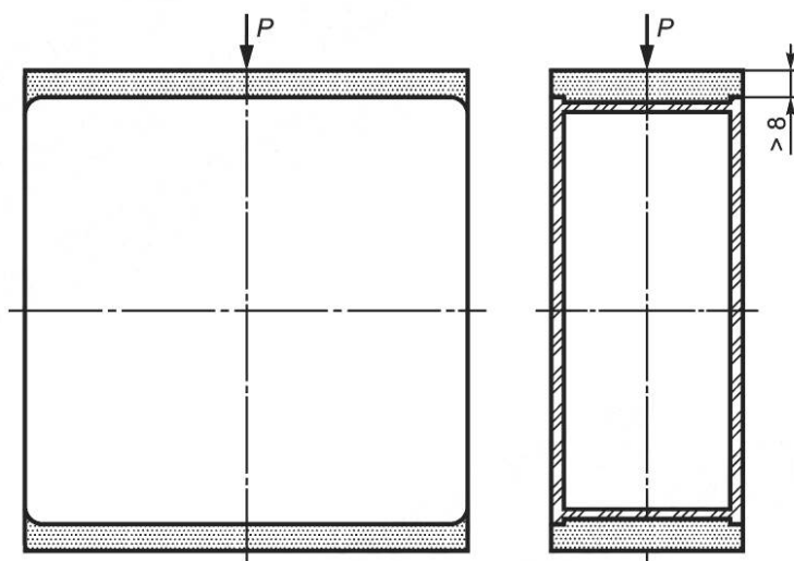
Рисунок 3 — Обмазка блока цементным раствором
