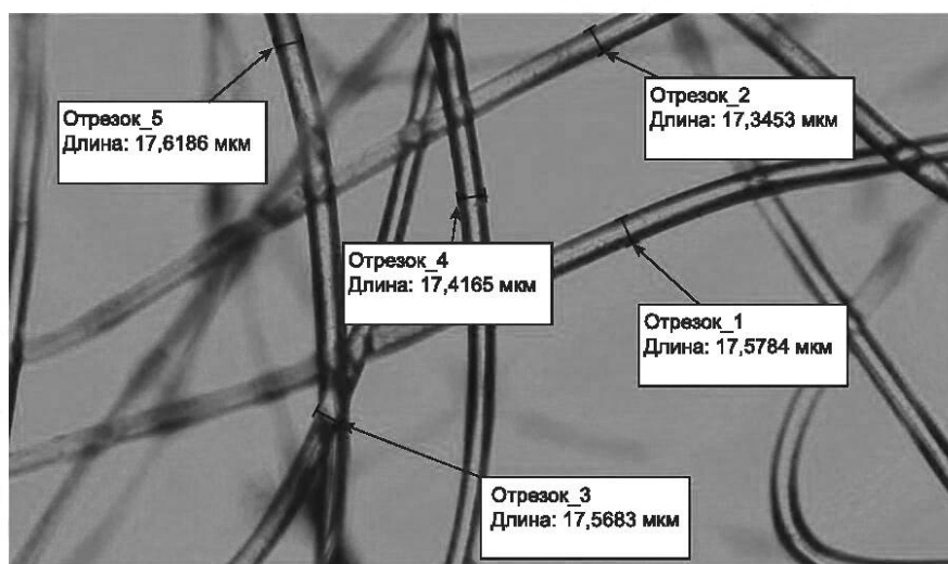
Рисунок А.3 — Пример измерения диаметра волокон с помощью программного обеспечения микроскопа
