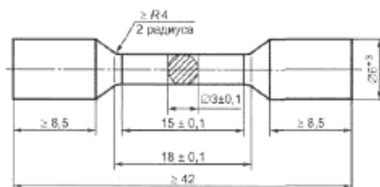
Рисунок 2 — Образец с удлиненной головкой
