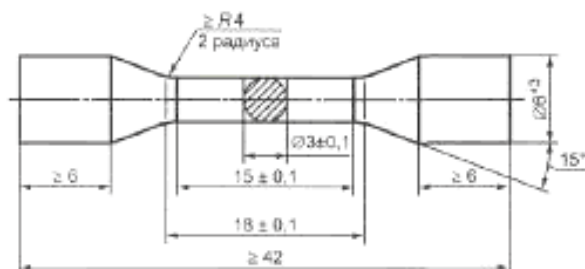
Рисунок 1 — Образец с короткой головкой
