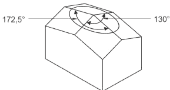
Рисунок 2 – Индентор Кнупа
