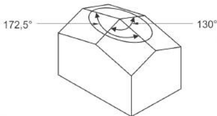
Рисунок 2 – Индентор Кнупа
