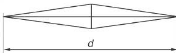
Рисунок 1 — Проекция отпечатка, полученного с помощью индентора Кнупа
