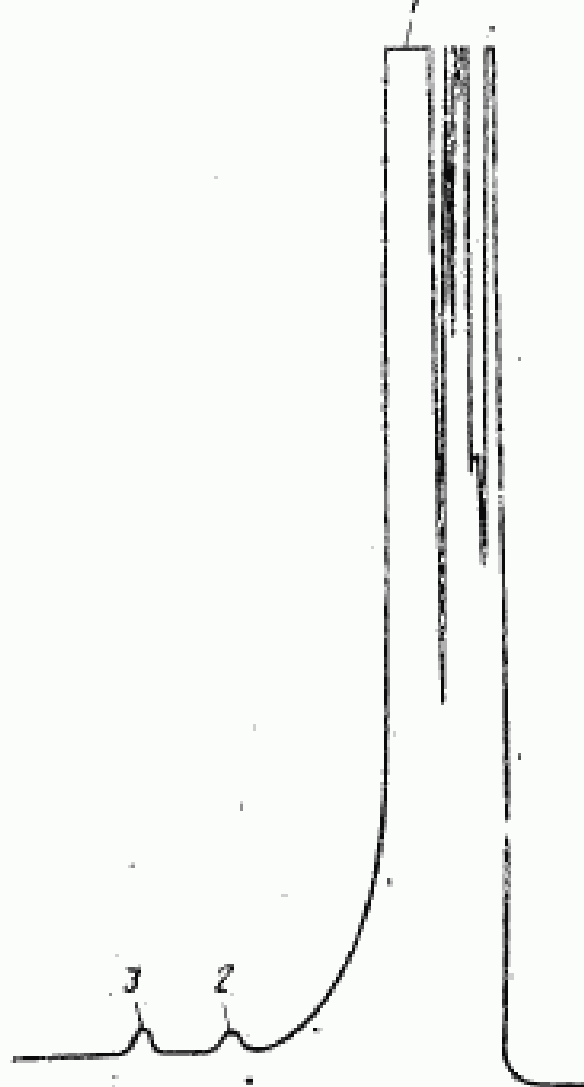
1—этилбензол; 2—диэтилбензол; 3— m -этил-изопропилбензол
