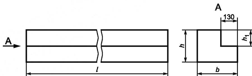
Рисунок 3 — Перемычка типа ПГ
