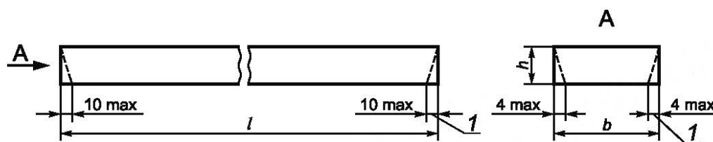
Рисунок 2 — Перемычка типа ПП
