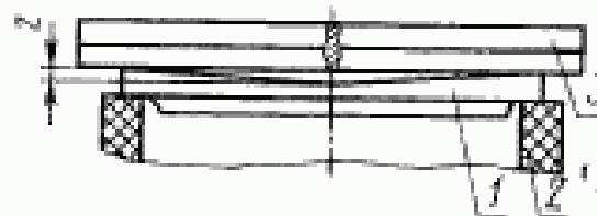
1—линза; 2—кольцевое гнездо; 3—до- верочная линейка
