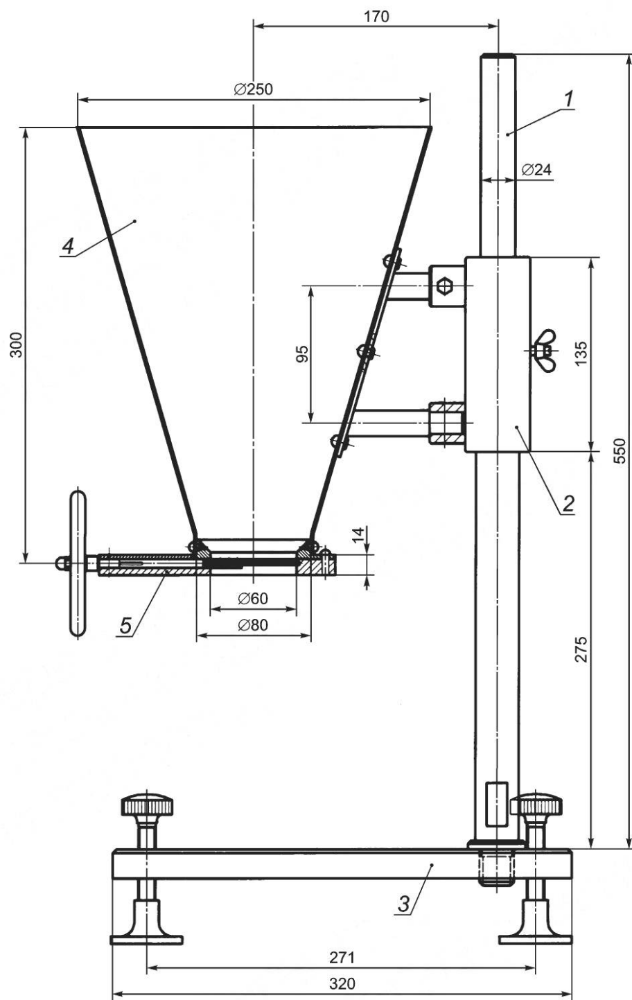
Рисунок 5 — Бункер для загрузки угля
