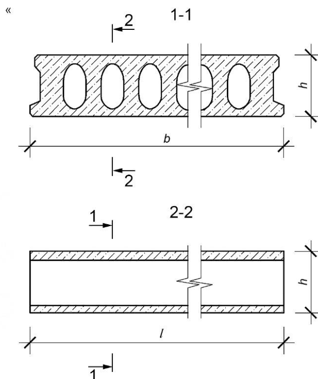
Рисунок 4 — Пример сечения плиты типа ПБ».
